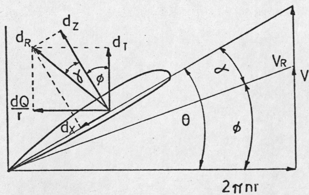
Fig. 1.2 Teoría de elementos de paleta
