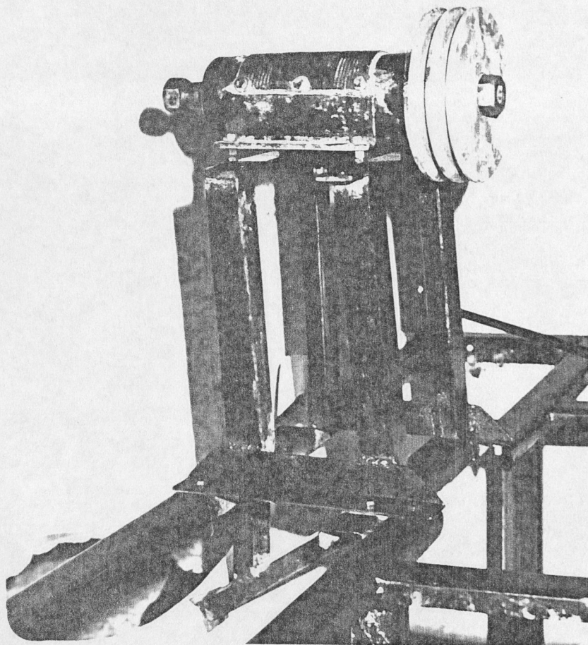
FOTO Nº 12.- Acople eje-polea
