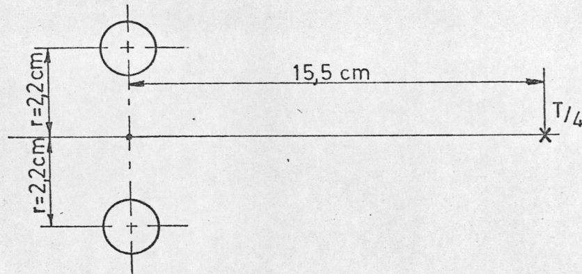
Fig.3-9. Centroide en los pernos de abrazadera.
