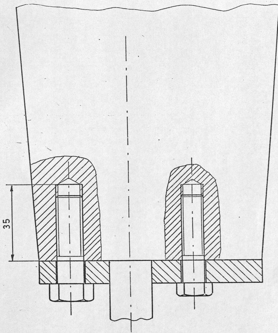
Fig. 3.5 Sujetadores de paleta
