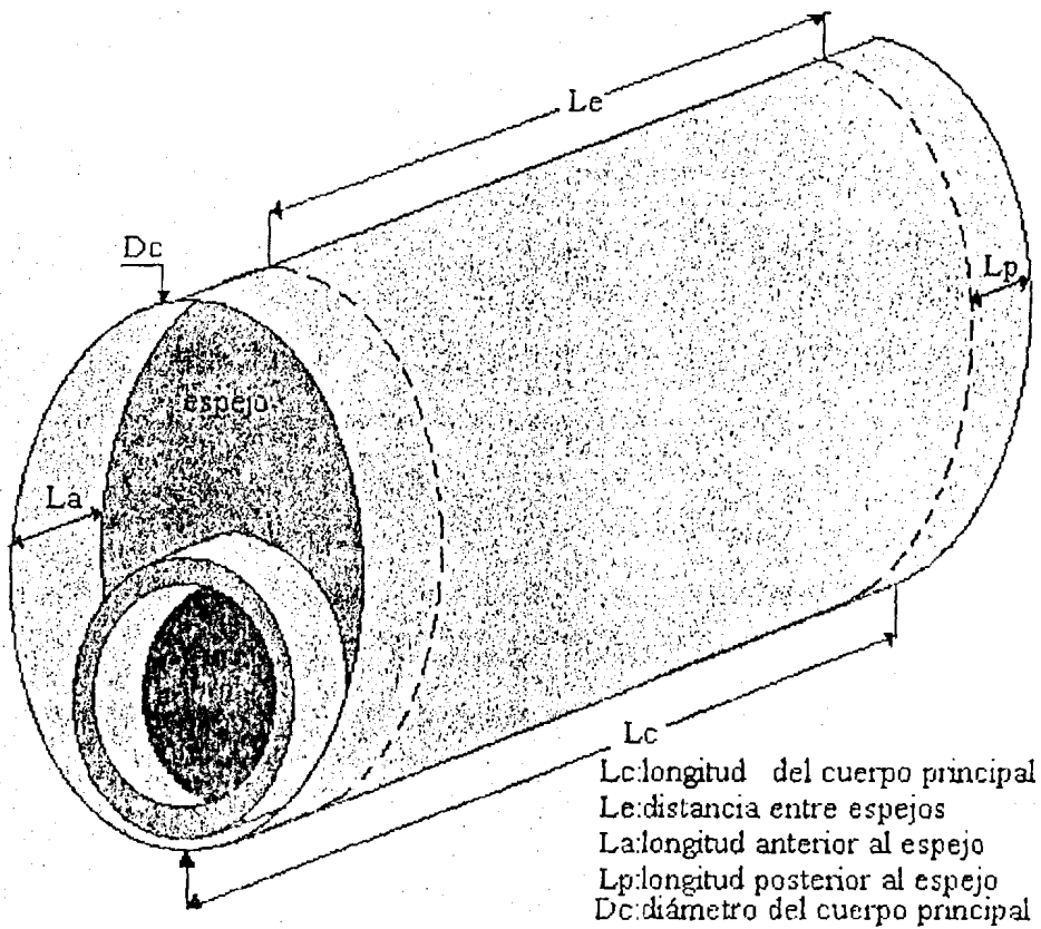
Fig. 3.4. Esquema de la Caldera.
