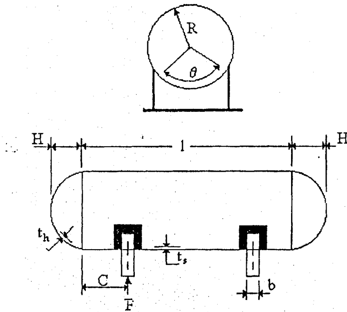
Fig. 2.9. Recipiente con silletas.
