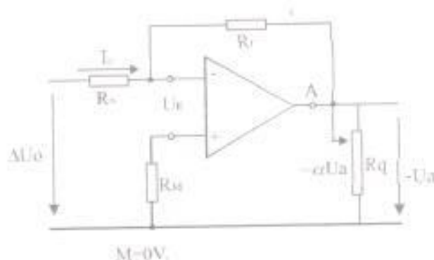
figura 2.3.- Elemento de acción proporcional (controlador P) con ganancia proporcional ajustable
