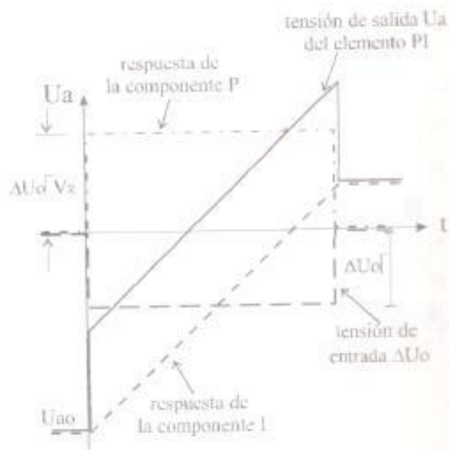
figura 2.5.-Resposta a un escalón ( U_a ) correspondiente a un elemento de acción proporcional e integral. En la figura se observa que esta respuesta está formada por la respuesta proporcional y por la respuesta integral que aparecen para una entrada en escalón \Delta U_0 de altura \Delta U_0 .
