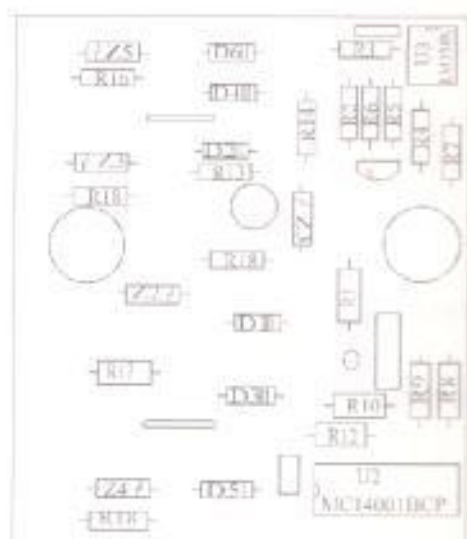
figura 4.3 Layout de la tarjeta de control
