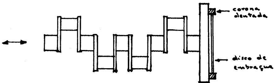
Fuga axial del cigueñal
