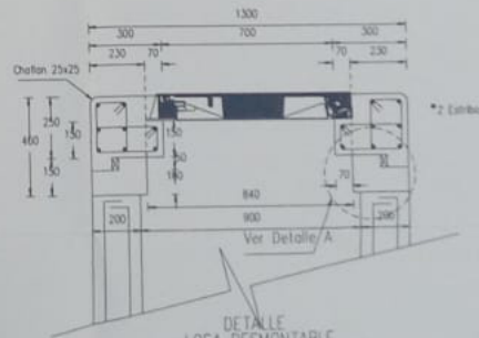
DETALLE LOSA DESMONTABLE Esc. 1 : 10
