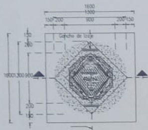
Esc. 1 : 20
