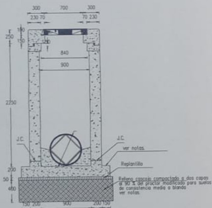
Esc. 1 : 20
