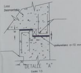
DETALLE "A" Esc. 1 : 5
