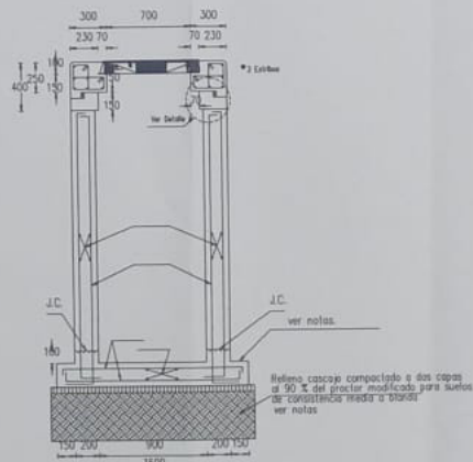
Esc. 1 : 20
