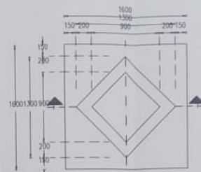
PLANTA Esc. 1 : 20
