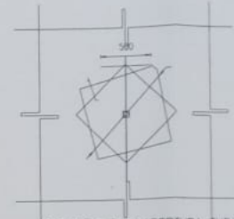
REFUERZO POR ABERTURA TUBO Esc. 1 : 20
