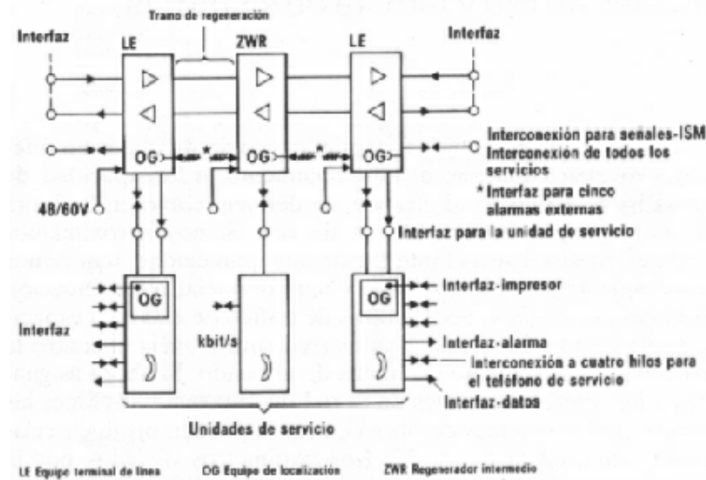
Fig. 1.8 Servicios suplementarios e interfaces
