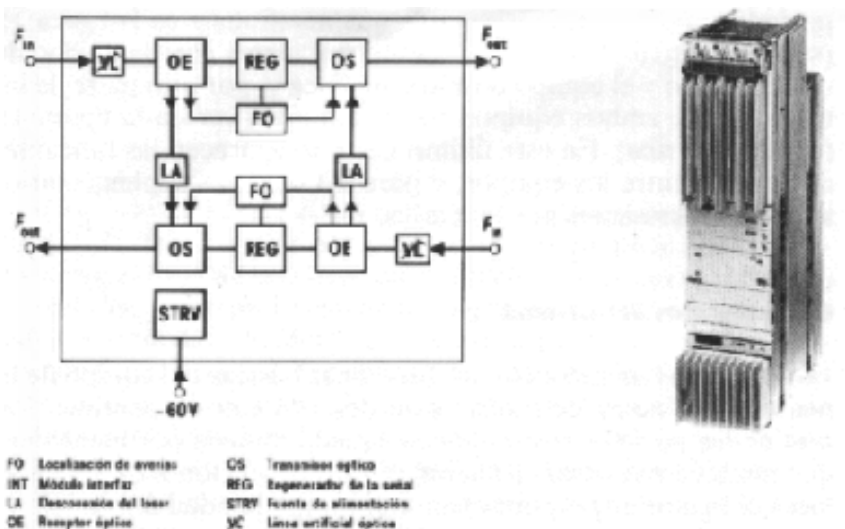
Fig. 1.5. Regenerador intermedio del sistema de transmisión por Fibras Ópticas
