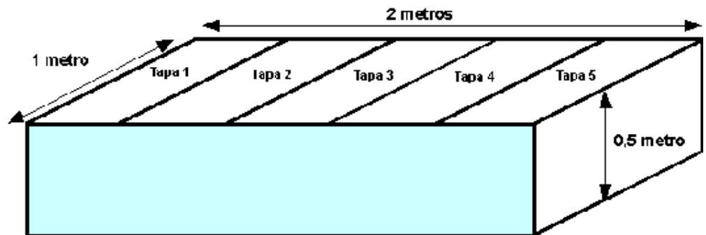
Figura 4.9. Cámara de protección de Fibra Optica enterrada.
