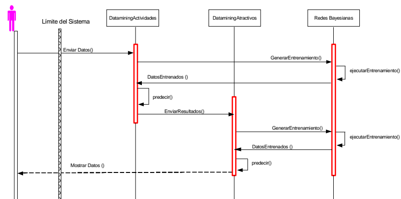
Figura 4.2. Sistema realiza búsqueda de sitios turísticos exitosamente
