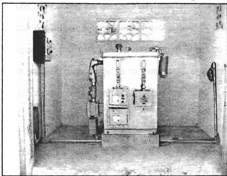
Figura 2.3 Rectificador Enfriado En Aceite, Tipo Antiexplosión
