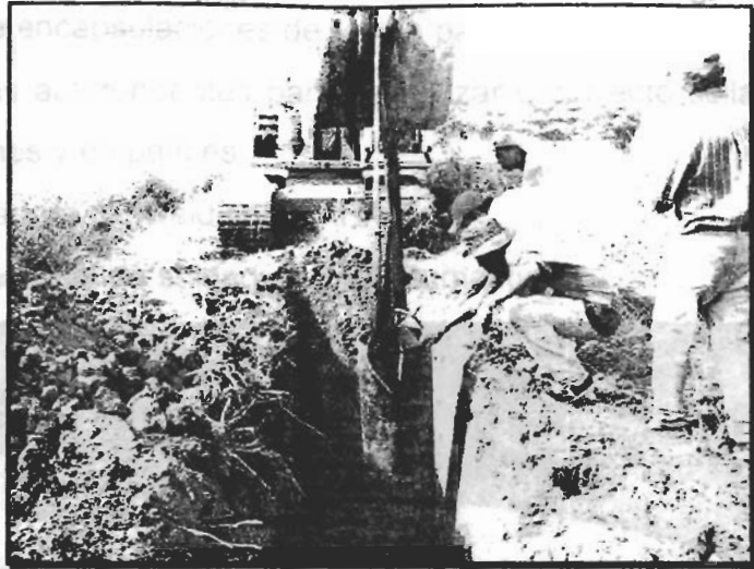
Figura 2.4 Instalación De La Cama De Ánodos
