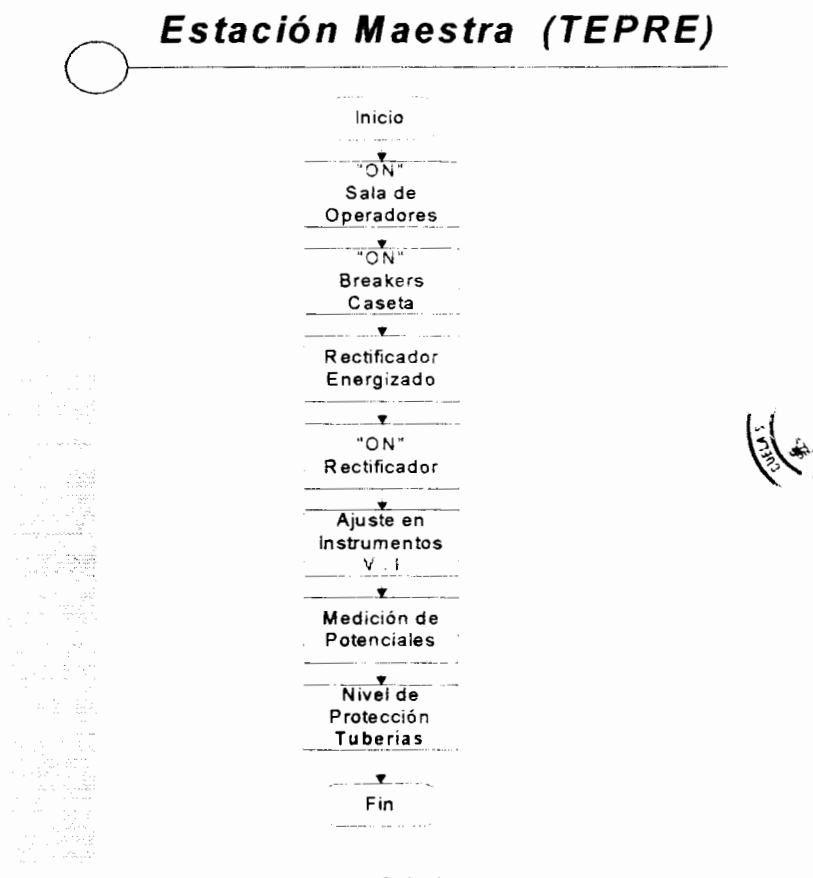
Figura 4.1 Diagrama De Proceso Del SPC
