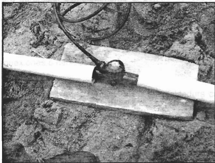
Figura 2.5 Encapsulación Epóxica Para Unión Y Sellado De Cables
