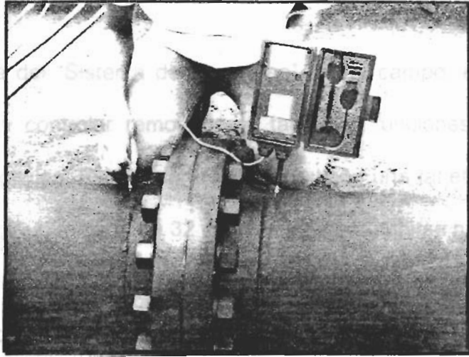
Figura 2.8 Medición De Aislamiento
