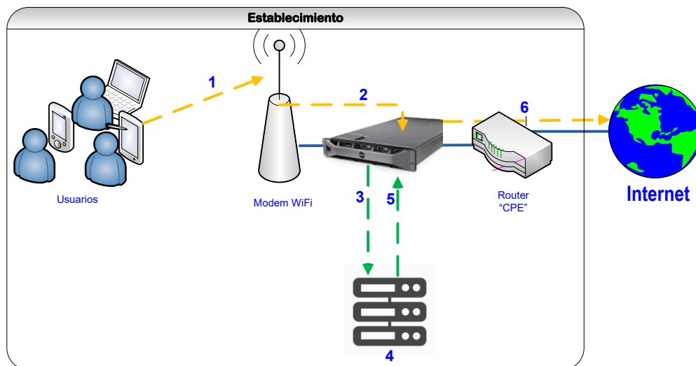
Figura 16: Proceso de control de navegación
