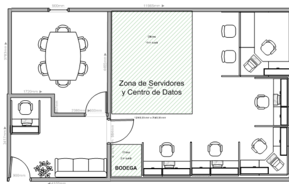
Figura 19: Oficina ControlNET
