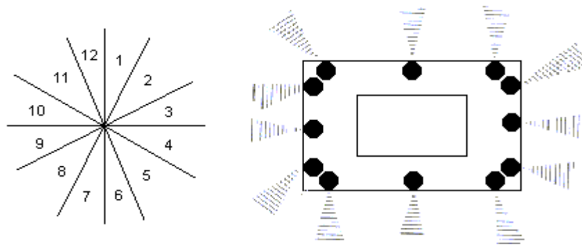
Figura 17. Configuración de 12 sectores
