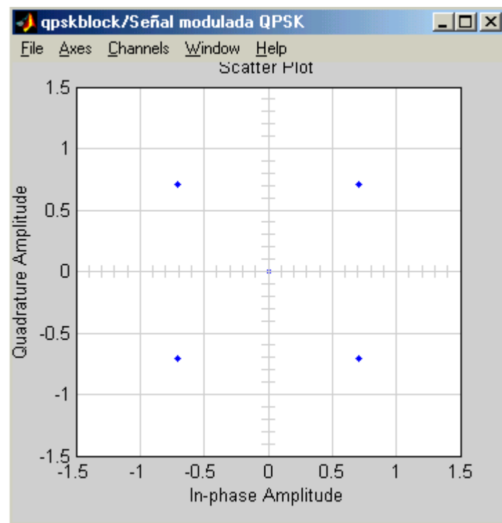
Figura 43. Constelación QPSK
