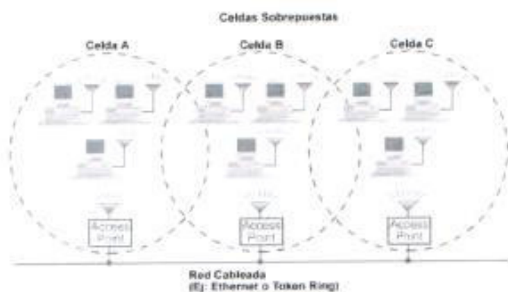
Gráfico 2- 16 Topología multiceldas[56]
