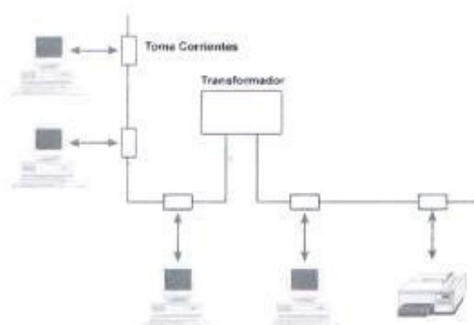
Gráfico 2-19 Esquema de transmisión de datos mediante energía eléctrica[59]
