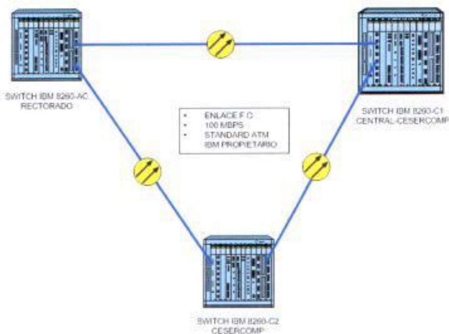
Gráfico 2-1 Esquema físico de la malla ATM[49]
