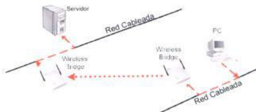
Gráfico 3-2 Configuración punto a punto usando el bridge inalámbrico [84]
