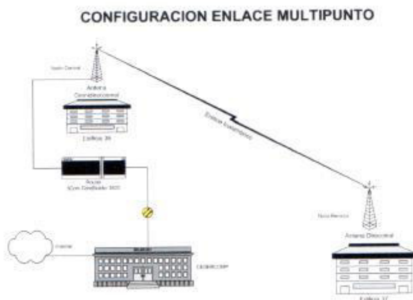
Gráfico 3-9 Esquema lógica del enlace multipunto
