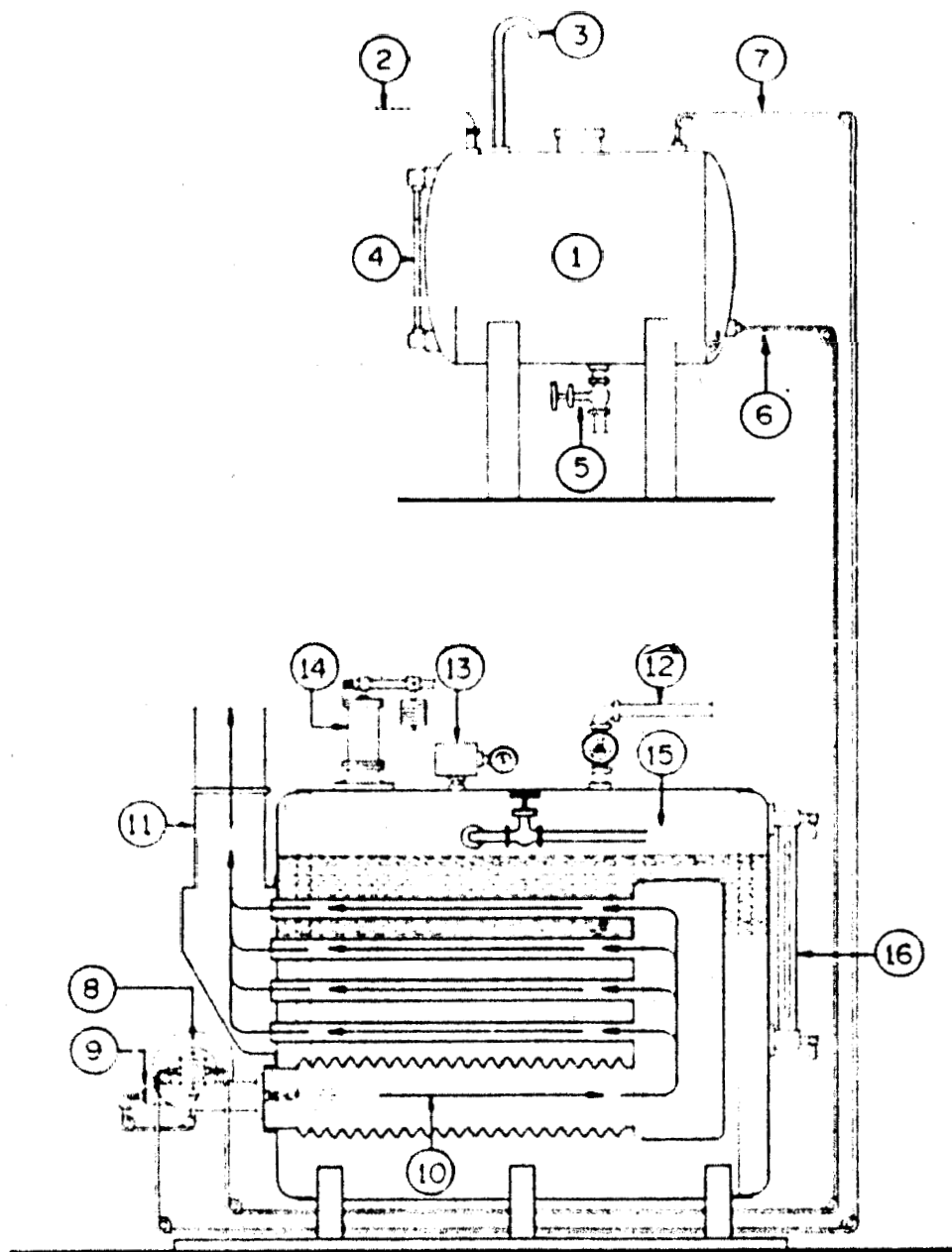
FIGURA 4.4. GENERADOR DE VAPOR
