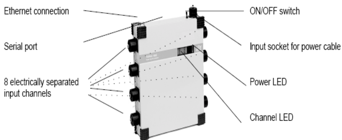
Figura 4.1.- Partes constitutivas del Analizador de Energía
