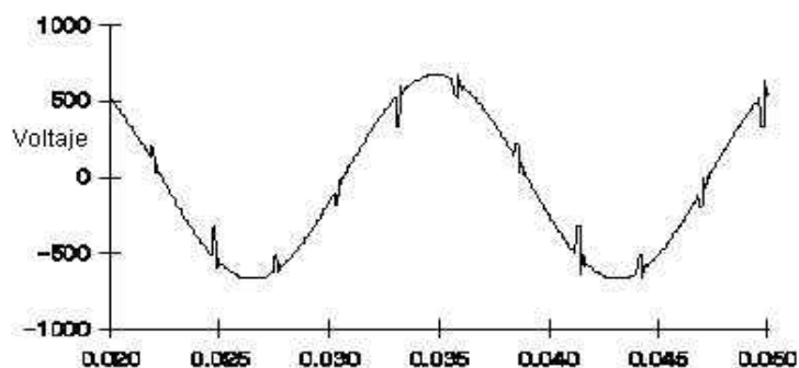
Figura 2.11.- Curva de espectro de corte
