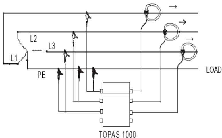
Figura 4.3.- Conexión Trifásica del Analizador de Energía Topas 1000
