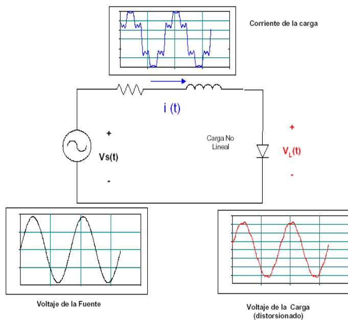
Figura 2.3 Distorsión de voltaje provocada por carga no lineal
