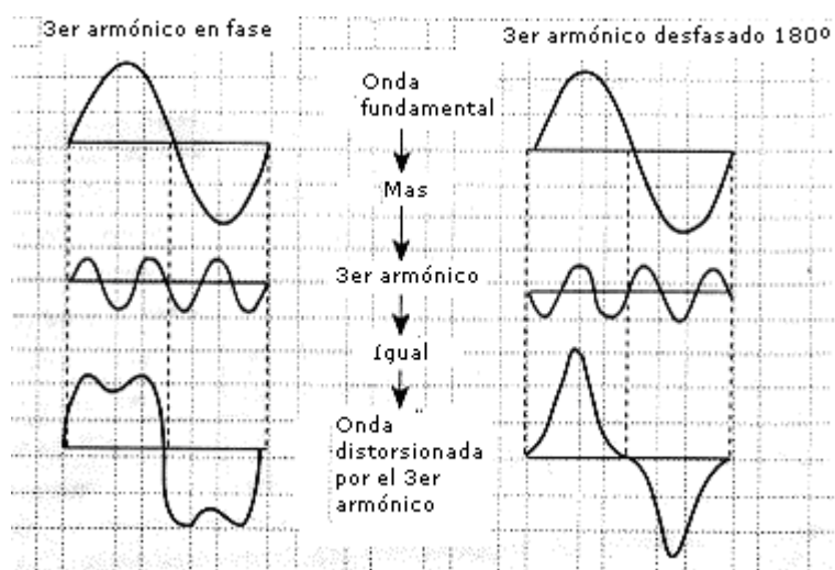
Figura 2.10.- Distorsión de una onda fundamental por armónicos
