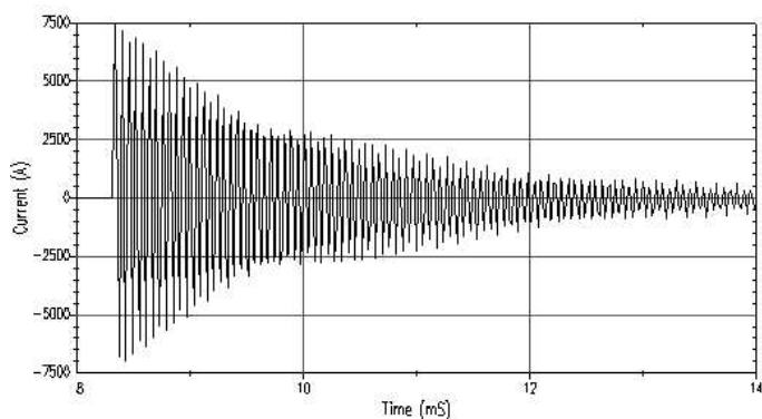
Figura 2.6.- Curva de espectro de transitorio oscilatorio
