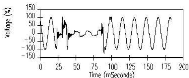
Figura 2.8.- Curva de espectro de sag
