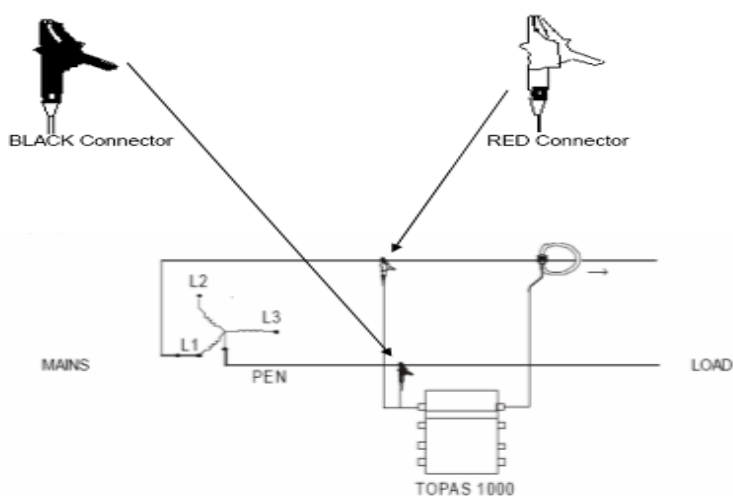
Figura 4.2.- Conexión Monofásica del Analizador de Energía
