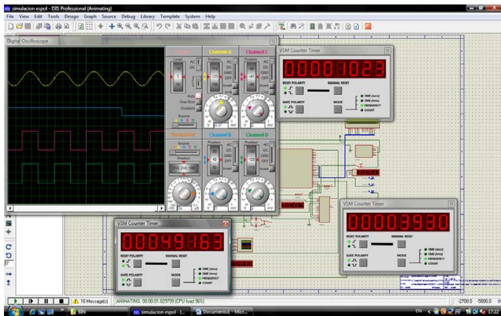
Figura 10: Frecuencia visualizada en osciloscopio y digitalmente
