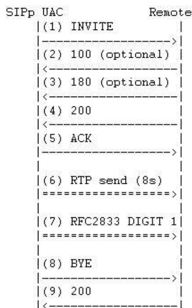
Figura 4-10 Escenario UAC con envío de flujo RTP
