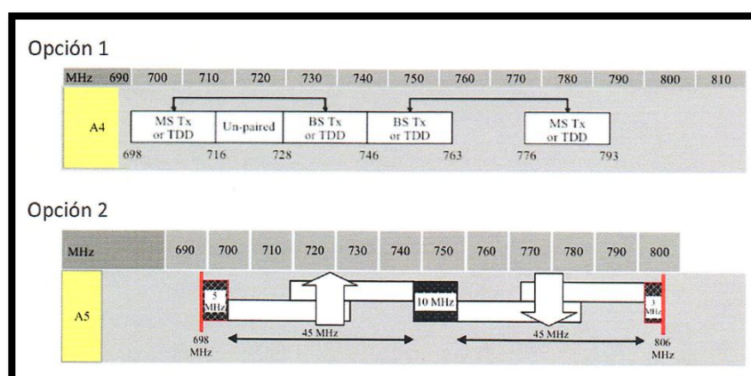
Figura 3.3 Recomendaciones para banda 698 a 806 MHz
