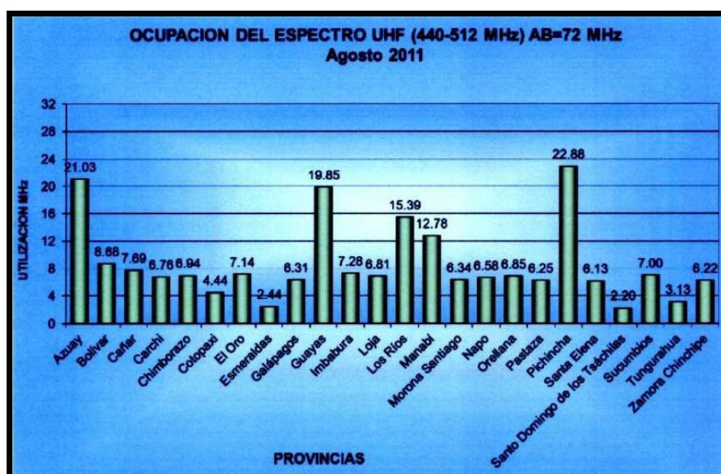
Figura 3.2 Ocupación del Espectro UHF por Provincias
