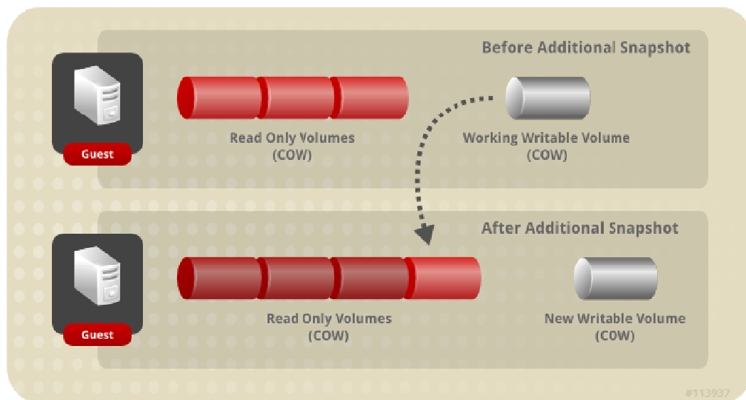
Figura 9: Snapshot
