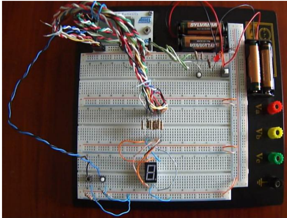
Figura 3.8. Circuito implementación del ejercicio 2 “Visualización en display desde 2 puertos alternados entre salida y alta impedancia”.
