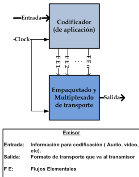
Figura 3.9 Transmisor
