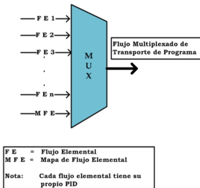
Figura 3.14 Multiplexado de transporte de programas
