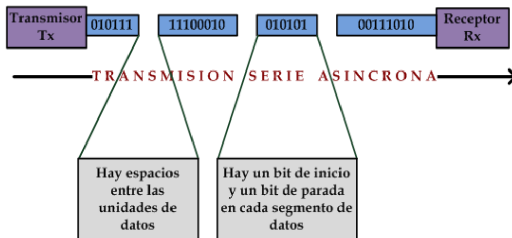
Figura 3.3 Transmisión Serie Asincrónica
