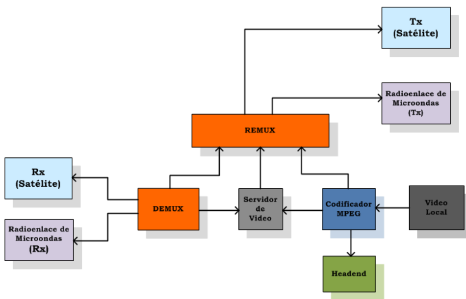
Figura 3.4 Esquema Transmisión y Recepción de una señal de televisión
