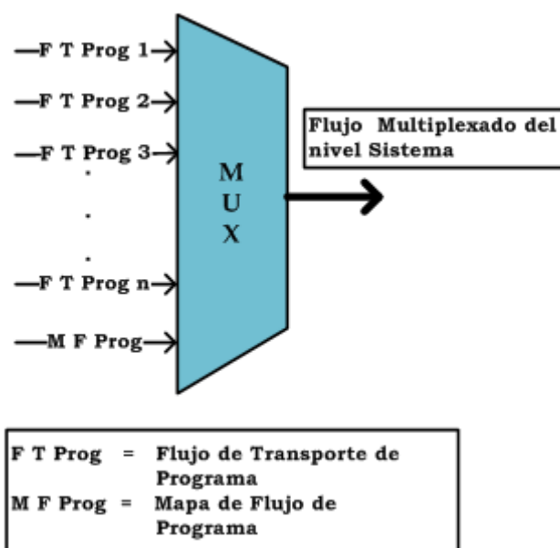
Figura 3.15 Multiplexado del Sistema
