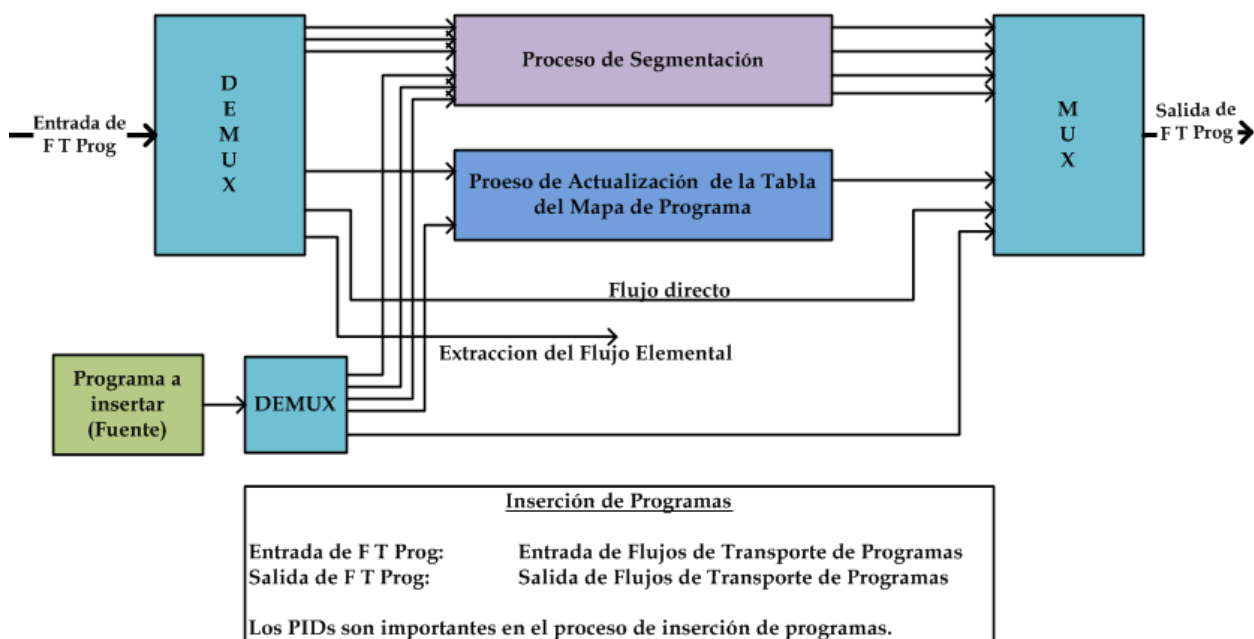
Figura 3.13 Proceso de Inserción de programas
