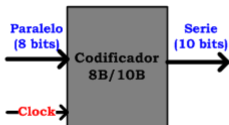
Figura 2.7 Codificador 8B/10B
