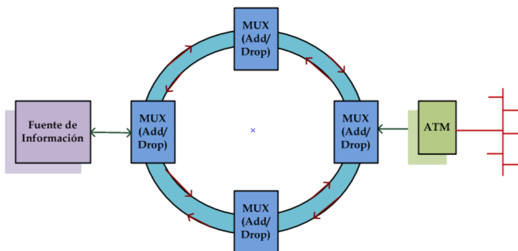
Figura 5.3 Topología anillo dual
