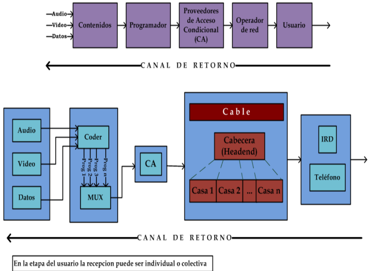
Figura 1.2 Modelo de Televisión Digital por Cable
