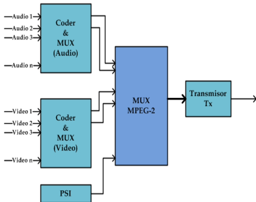
Figura 1.5 Cadena de Transmisión
