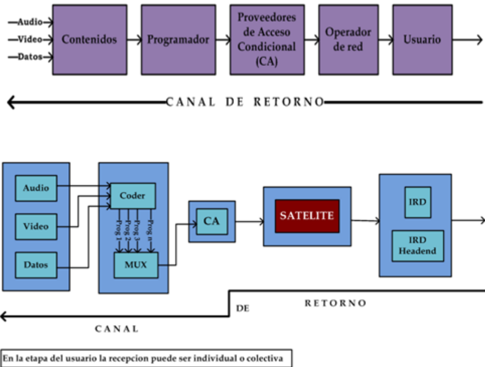
Figura 4.1 Modelo de Televisión Digital por Satélite
