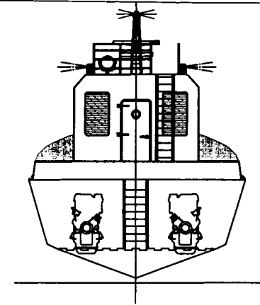
VISTA TRANSVERSAL
