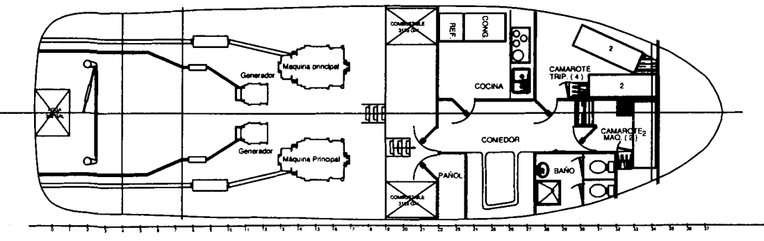
CUBIERTA 200
