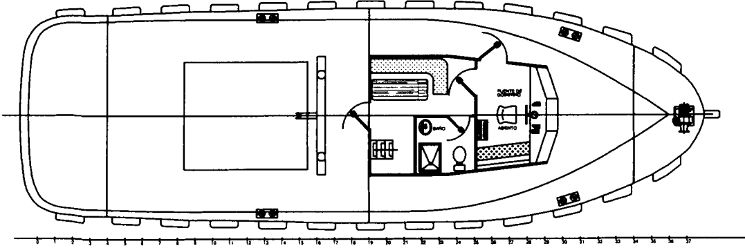
CUBIERTA 100
