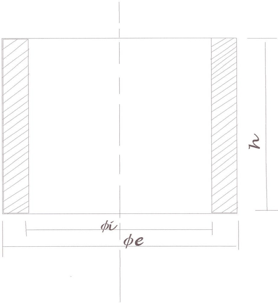
FIG. 1 COJINETE RADIAL
