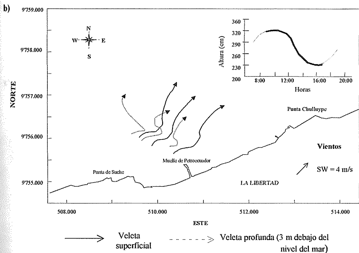
Figura 2.10. Trayectoria seguida por las veletas en la cuadratura de octubre/94. En a) y b), las mediciones fueron realizadas en refluo.
