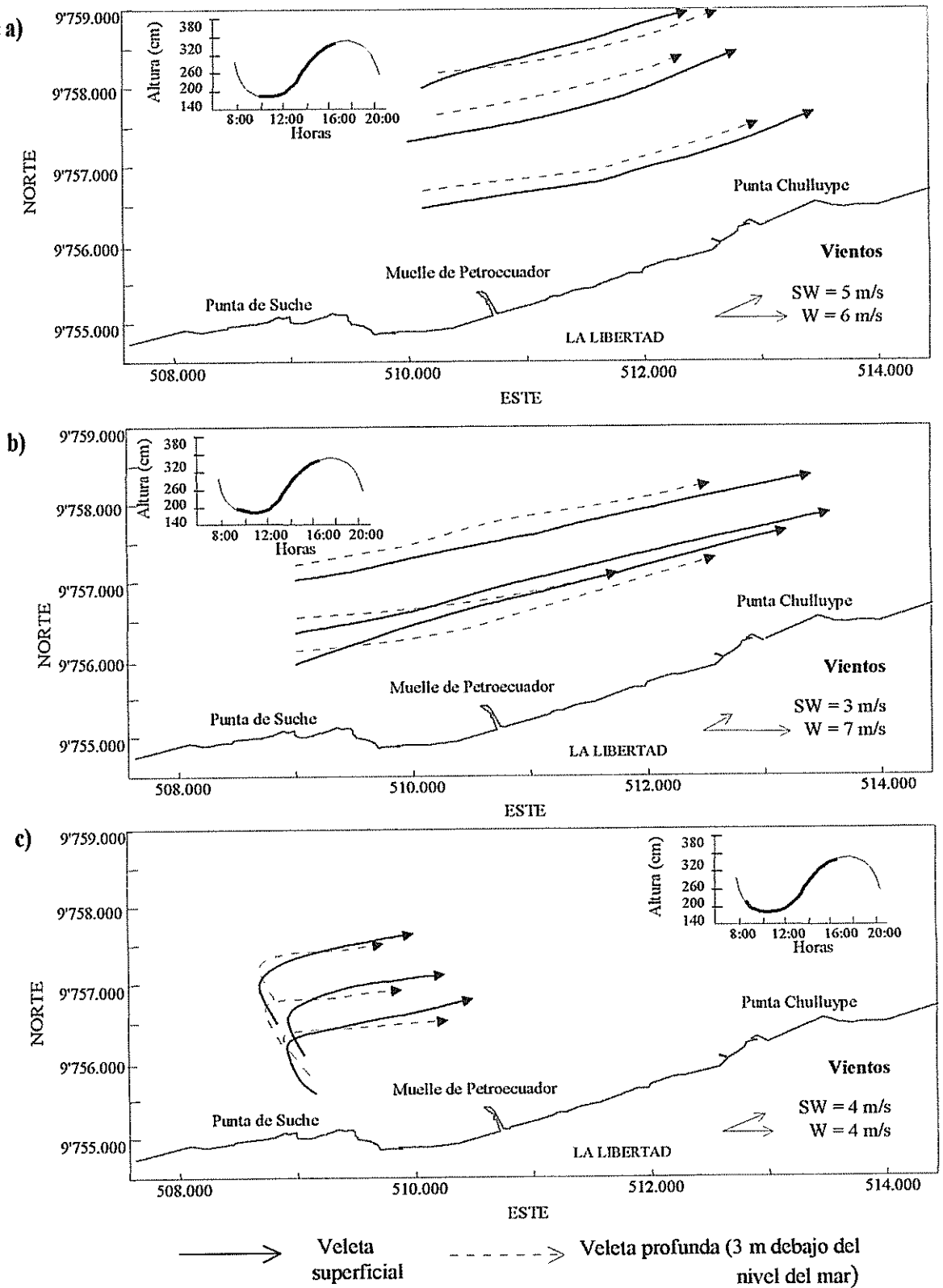
Figura 2.11. Trayectoria de las veletas en la sicigia de octubre/94. En a) y b), las mediciones corresponden al flujo, y en c), a las dos fases de marea.
