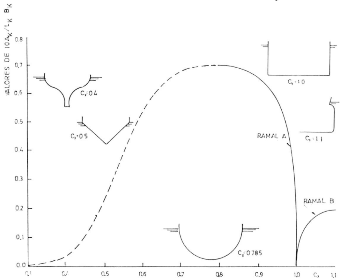
CURVA PARA DETERMINAR EL AREA DE QUILLA DE BALANCE FIGURA No 4.5
