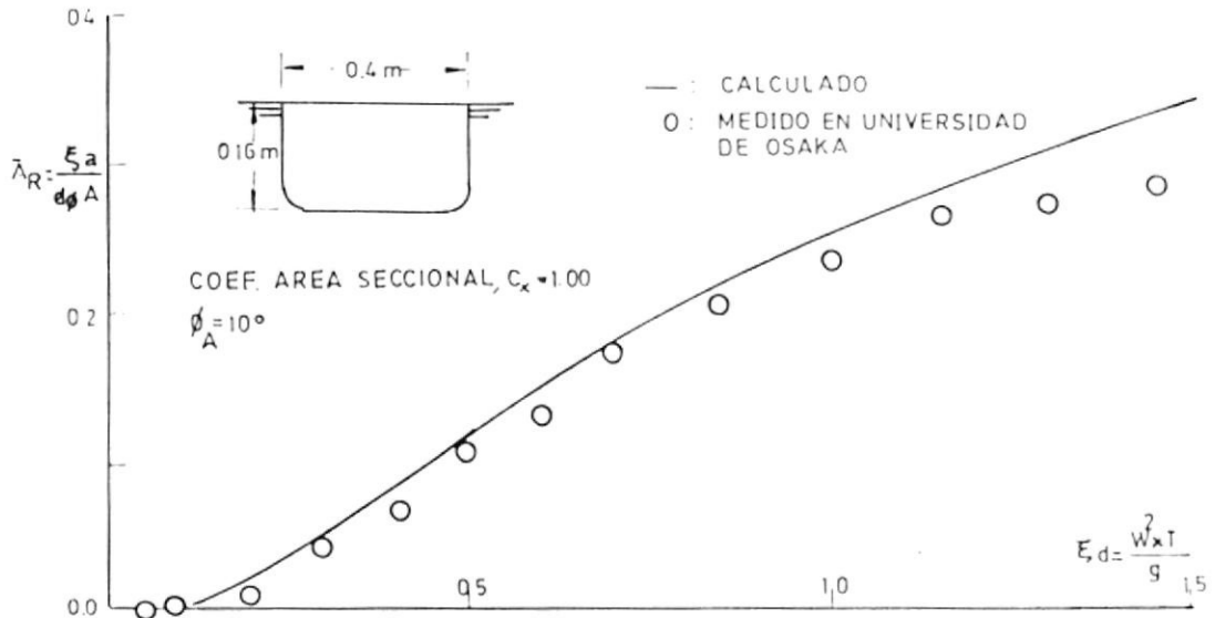
AMPLITUD DE LA OLA RADIADA POR EL CILINDRO CON FORMAS DE LEWIS REF. (25)
