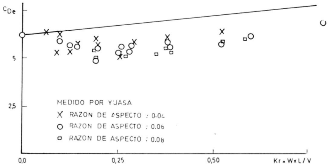
EFFECTO DE LA VELOCIDAD DE AVANCE EN EL COEFICIENTE DE ARRASTRE DE LA QUILLA DE BALANCE
