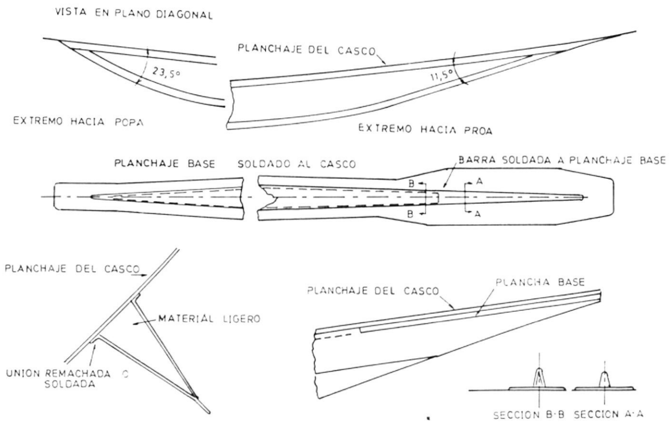
ARREGLO ESTRUCTURAL DE LA QUILLA DE BALANCE FIGURA No 4.6
