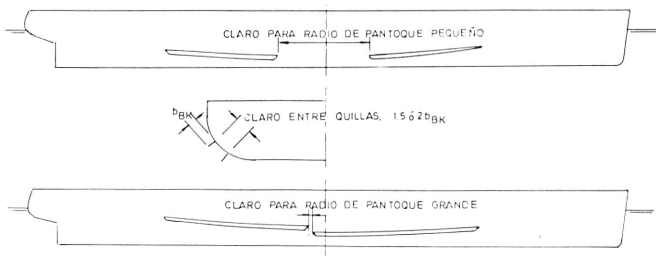
DISPOSICION LONGITUDINAL CON CLAROS DE QUILLAS DE BALANCE FIGURA No 43
