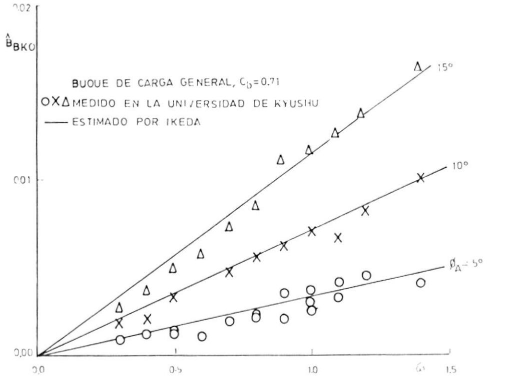
EFFECTO DE LA QUILLA DE BALANCE EN EL COEFICIENTE DE AMORTIGUAMIENTO PARA UN NUMERO DE FROUDE IGUAL A CERO REF. (25) FIGURA No. 3, 10
