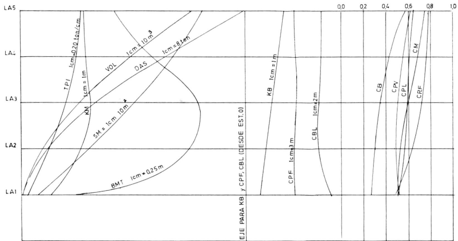
CURVAS HIDROSTATICAS LANCHAS DE PESCA ARTESANAL FIGURA No. B7
