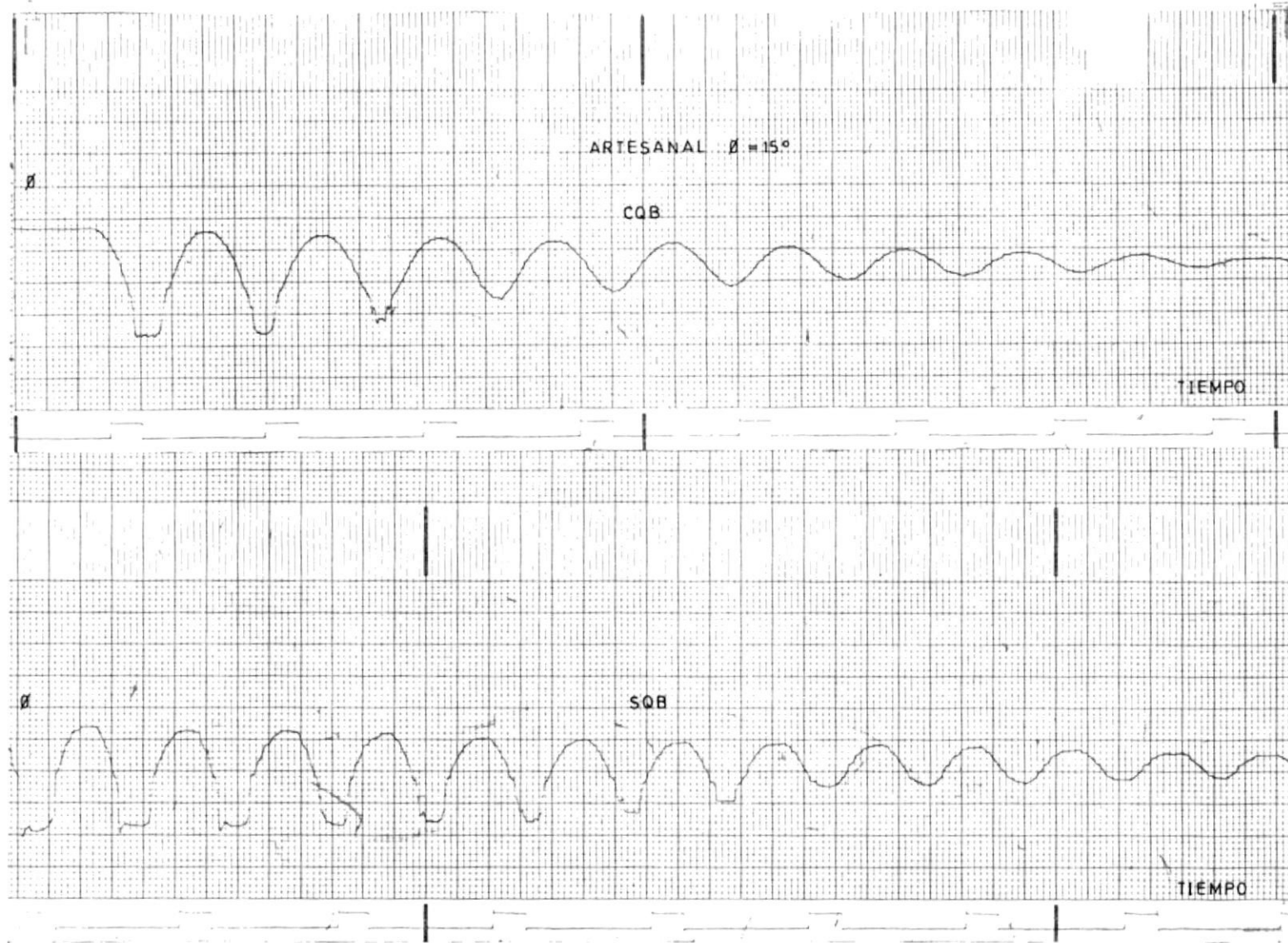
CURVA DE EXTINCION DEL MOVIMIENTO DE ROLIDO: FIGURA No. B.14
