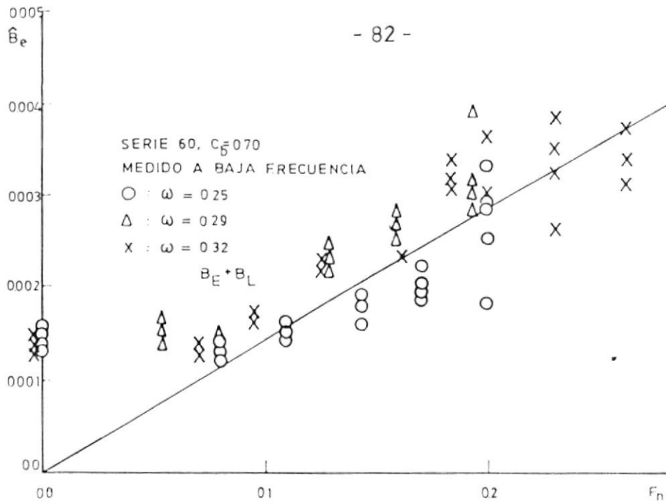
ADICION DE LAS COMPONENTES POR REMOLINOS Y SUSTENTACION EN PRUEBAS FORZADAS DE ROLIDO
