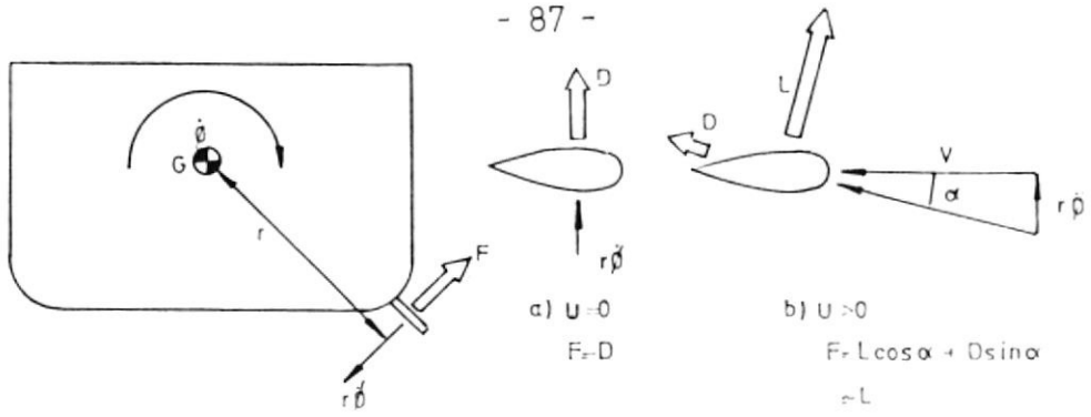
AMORTIGUAMIENTO EN ROLIDO DEBIDO A SUPERFICIES DE SUSTENTACION
