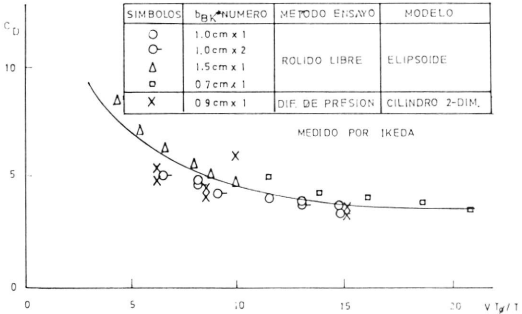
COEFICIENTE DE ARRASTRE DEBIDO A QUILLA DE BALANCE REF. (25)
