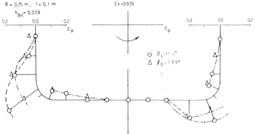
DISTRIBUCION DE LA PRESION EN EL CASO INDUCIDA POR LA QUILLA DE BALANCE FIGURA No. 3, 9
