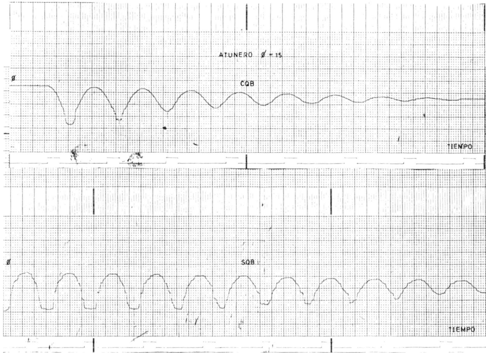
CURVA DE EXTINCION DEL MOVIMIENTO DE ROLIDO FIGURA No B.15
