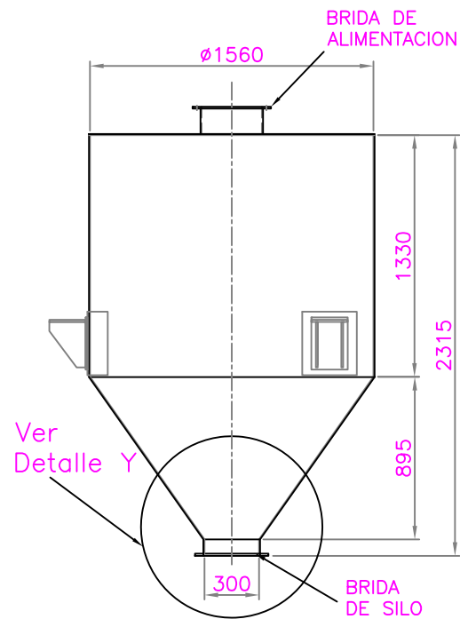
SILO S2 PARA ARENA \phi 1560mm ESCALA 1 : 40
