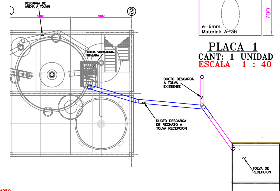
VISTA EN PLANTA-DESCARGA DE CHUTE ESCALA 1 : 150
