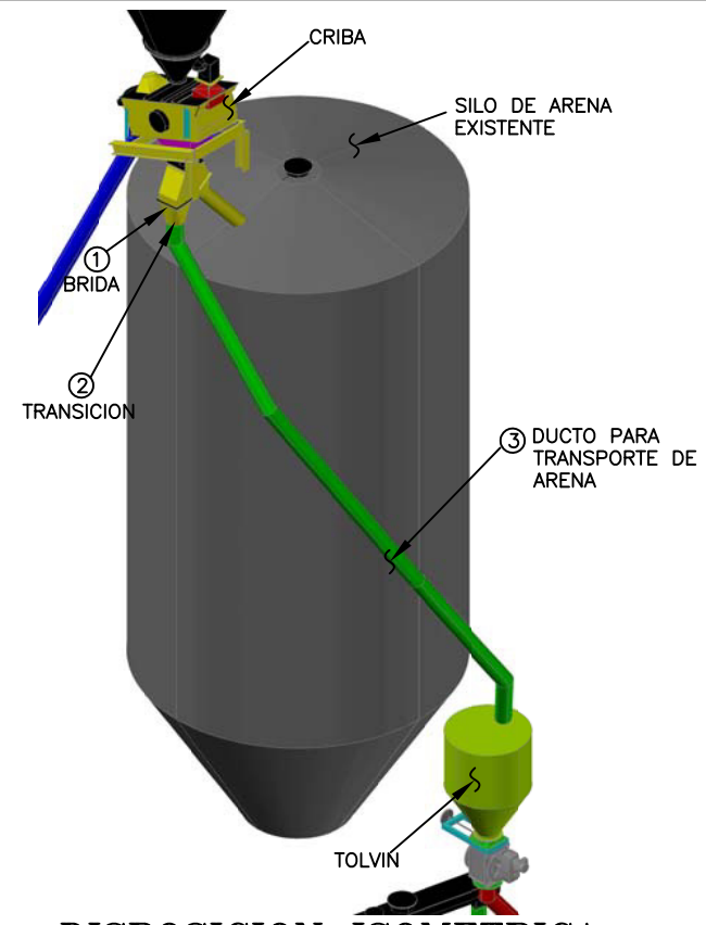
DISPOSICION ISOMETRICA
