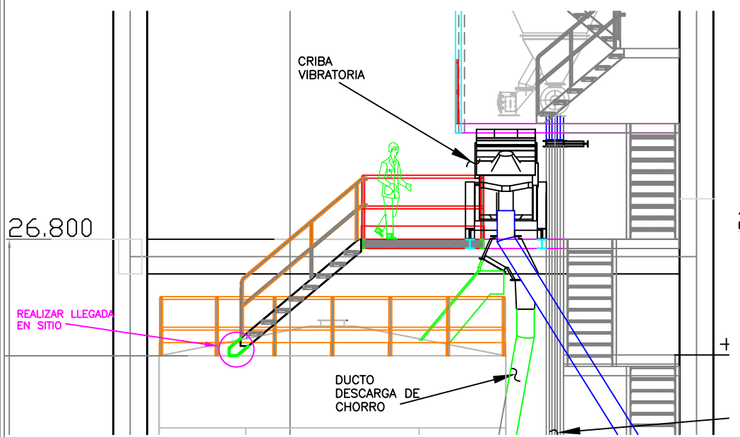
VISTA FRONTAL ESCALA 1 : 100
