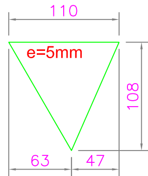
PLACA P4 (Cant. 8) ESCALA 1 : 4
