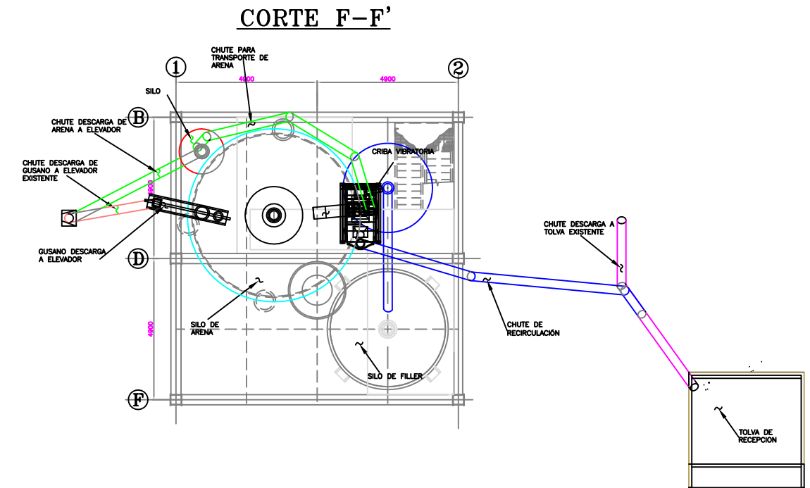
PLANTA NIVEL + 28.800
