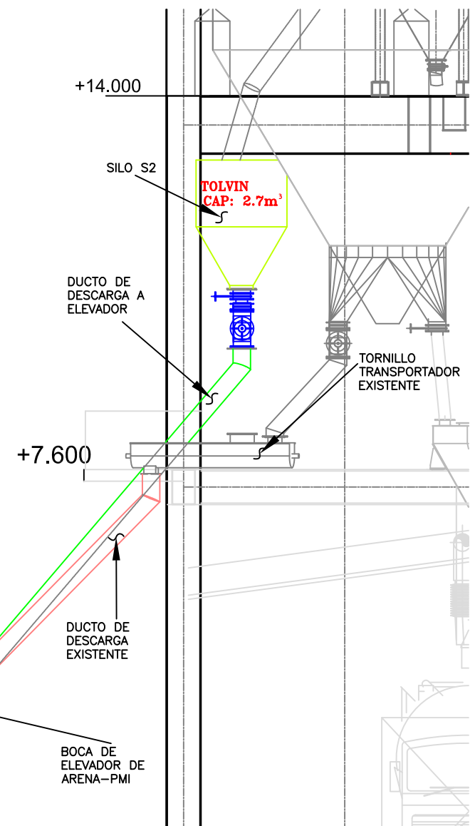
VISTA FRONTAL DESCARGA ELEVADOR ESCALA 1 : 100
