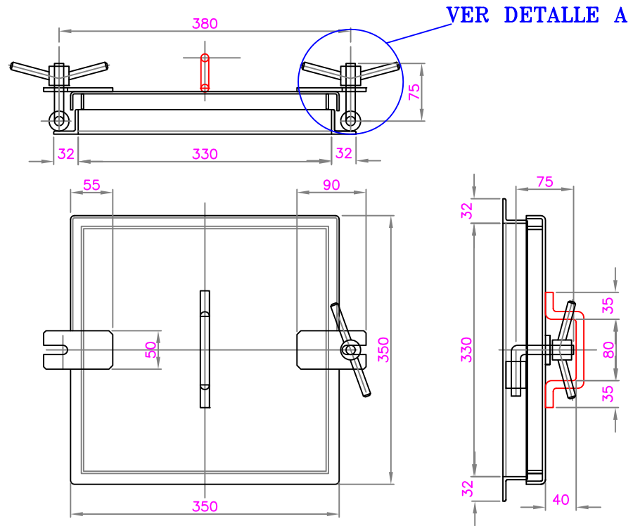
TAPA DE INSPECCION ESCALA 1 : 2,5
