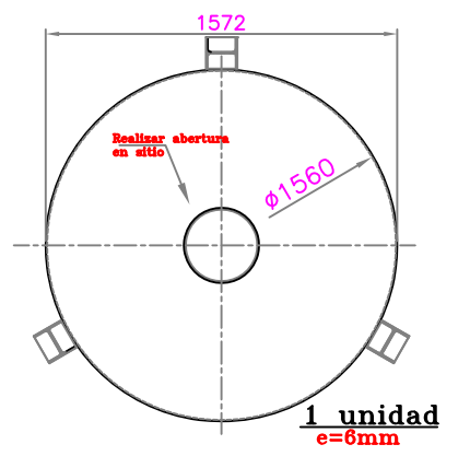
TAPA DE SILO
