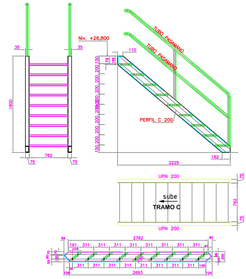
DETALLE DE ESCALERA ESCALA 1 : 75
