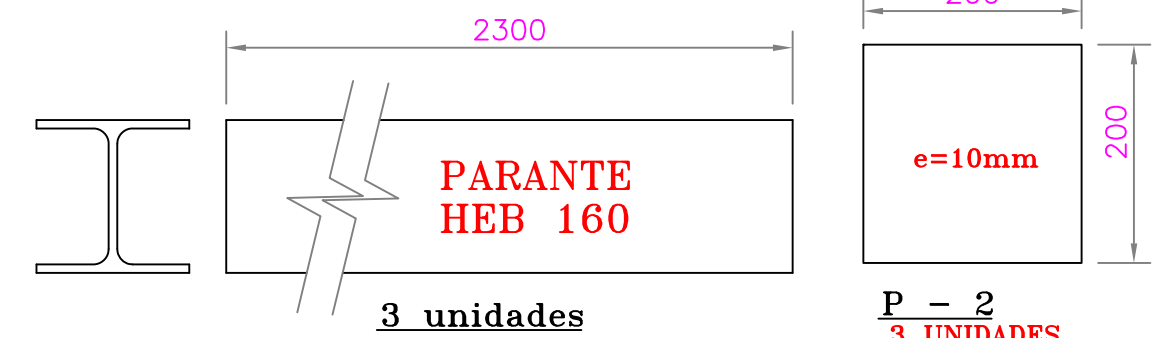
DETALLE DE SOPORTES
