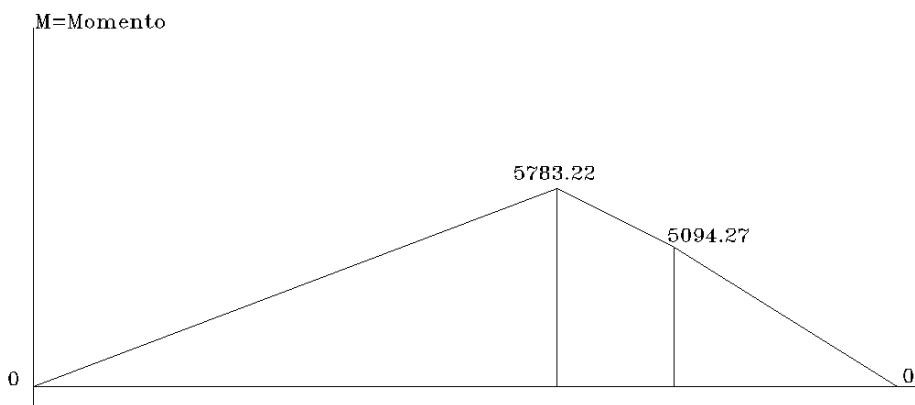
FIGURA 3.10 - DIAGRAMA DE MOMENTO.
