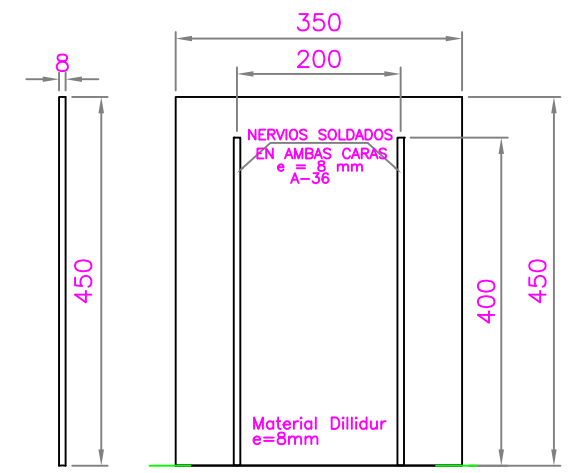
ITEM 8 (Cant. 1u) ESCALA 1 : 10
