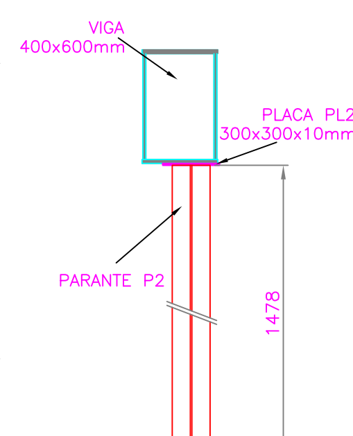
SOPORTE PARANTE P2 CANT: 1 UNIDAD ESCALA 1 : 30
