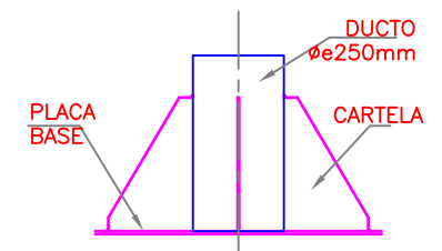
DISPOSICION DE CARTELAS ESCALA 1 : 25
