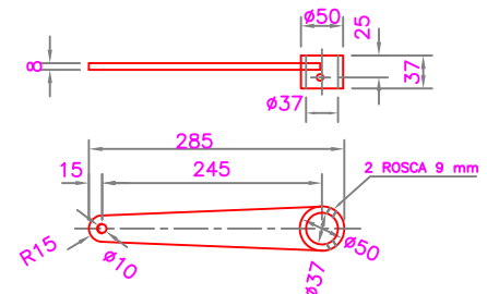
ITEM 3 (Cant. 1u) ESCALA 1 : 10
