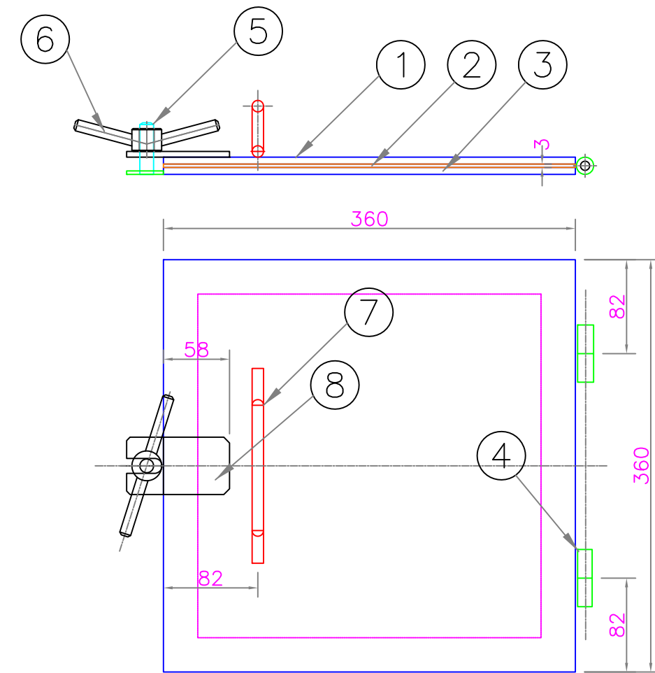
DISPOSICION DE TAPA ESCALA 1 : 5
