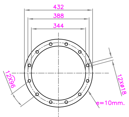
BRIDA DE ALIMENTACION
