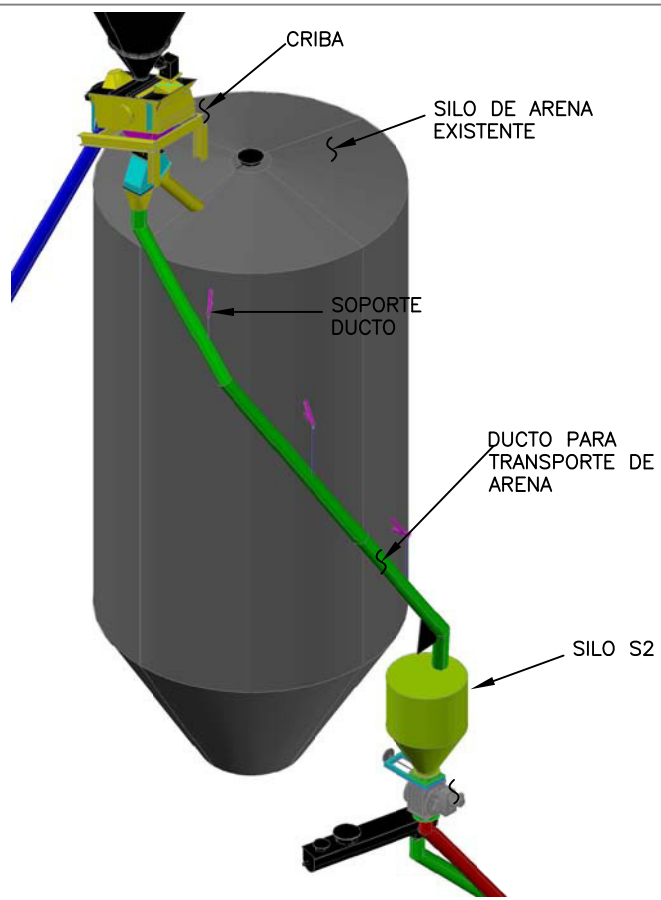
DISPOSICION ISOMETRICA
