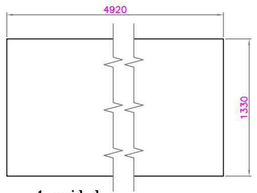
DESARROLLO DE CUERPO Y CONO
