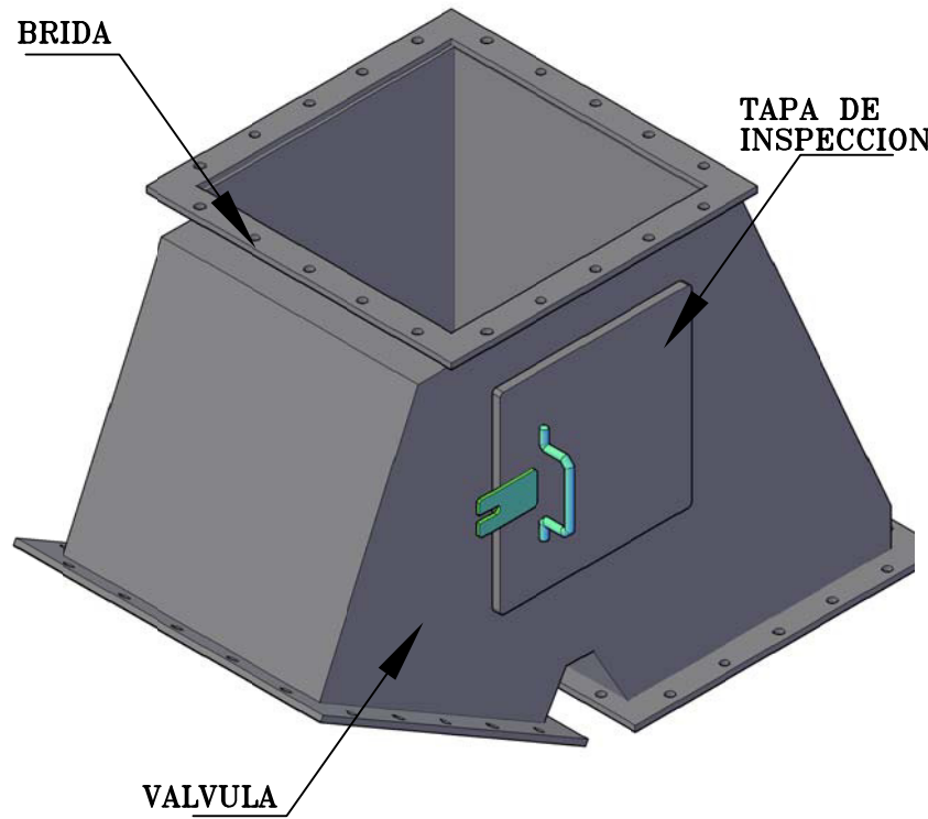
VISTA ISOMETRICA DE VALVULA DE DOS VIAS ESCALA 1 : 7.5
