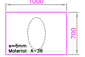
PLACA 1 CANT: 1 UNIDAD ESCALA 1 : 40
