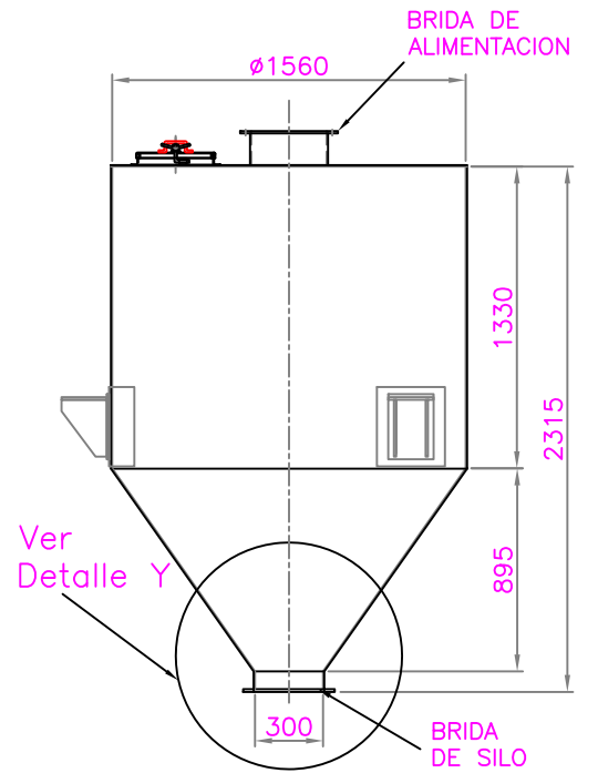
SILO S2 PARA ARENA \phi 1560mm ESCALA 1 : 40
