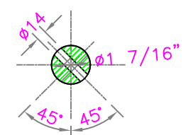
CORTE A-A' ESCALA 1 : 7.5
