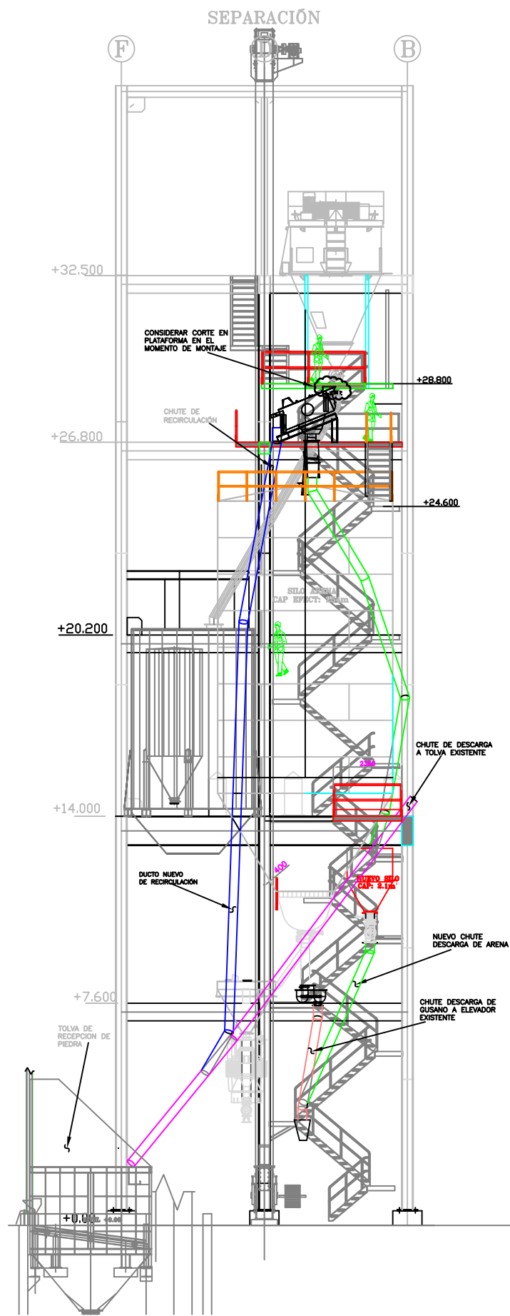
VISTA LATERAL
