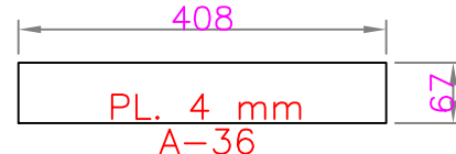
ITEM 13 (Cant. 1u) ESCALA 1 : 10
