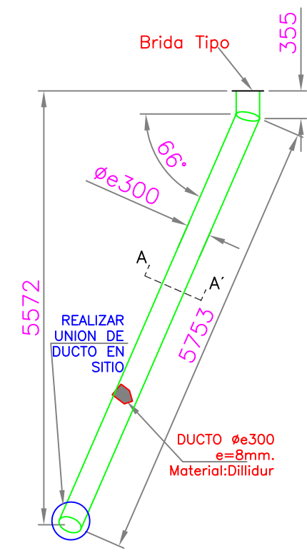
VISTA LATERAL DEL DUCTO ESCALA 1 : 75
