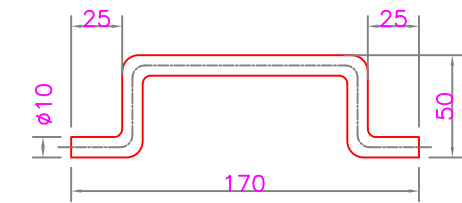
7 MANIJA (Cant. 1u) ESCALA 1 : 4
