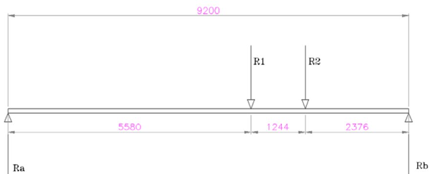
FIGURA 3.7 - DIAGRAMA DE FUERZAS.
