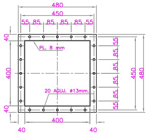
BRIDA-ITEM 1 (Cant. 3u) ESCALA 1 : 15
