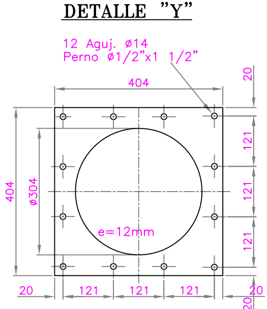
BRIDA DE SILO
