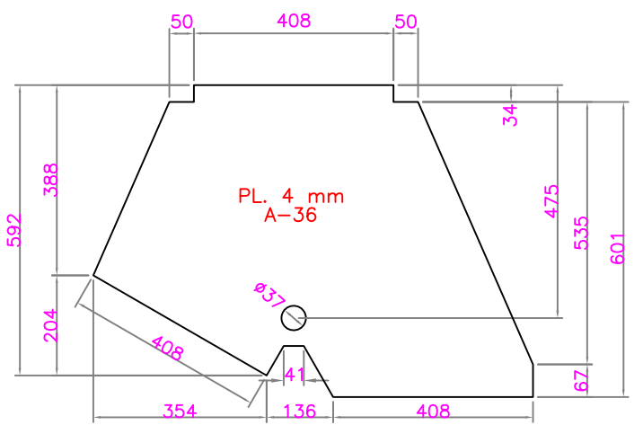
ITEM 2 (Cant. 2u) ESCALA 1 : 15
