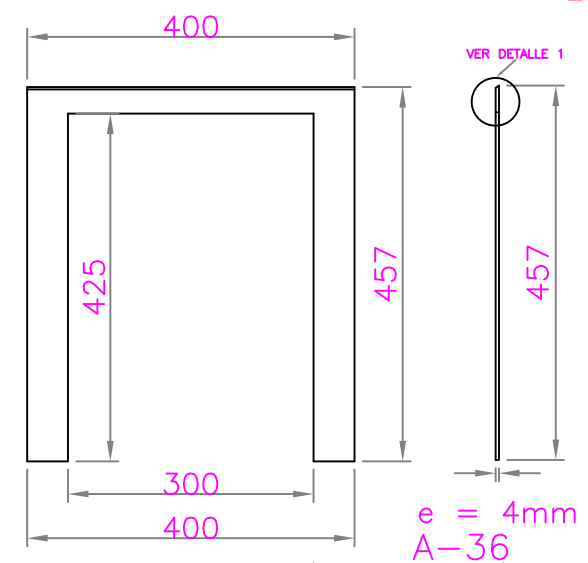
ITEM 7 (Cant. 2u) ESCALA 1 : 10
