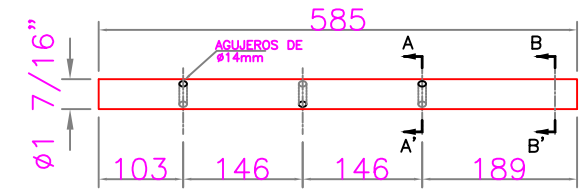
EJE \phi 1 7/16" (Cant: 1u) ESCALA 1 : 10
