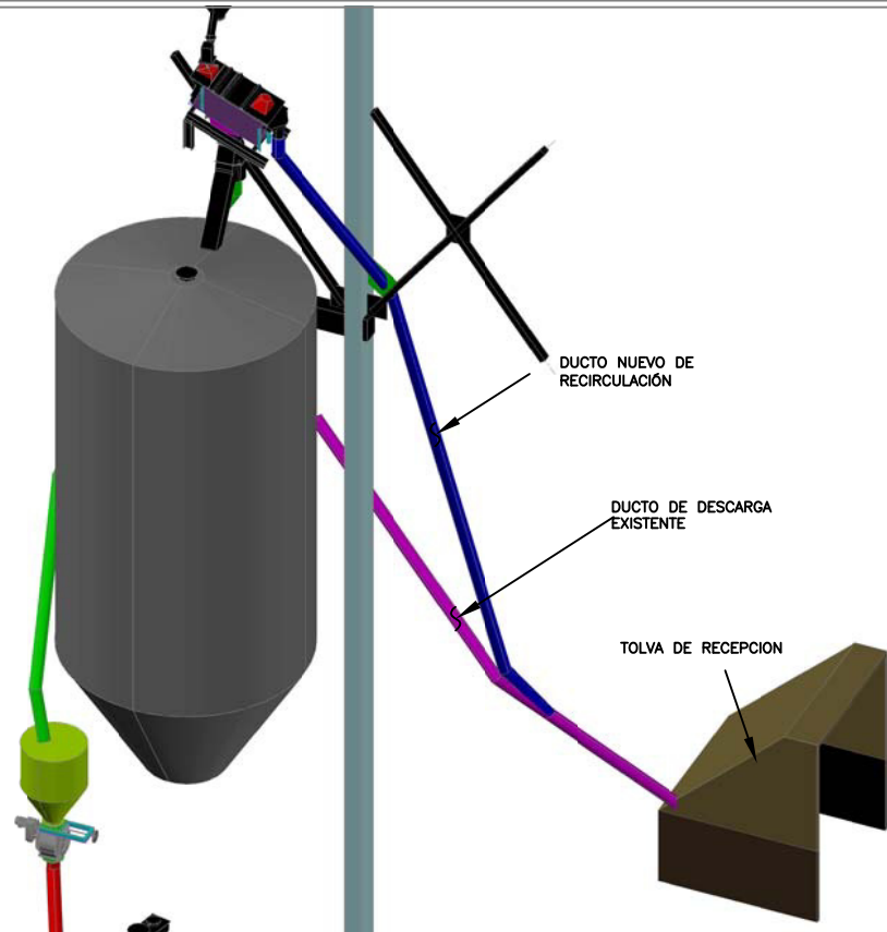
DISPOSICION ISOMETRICA L=26000mm
