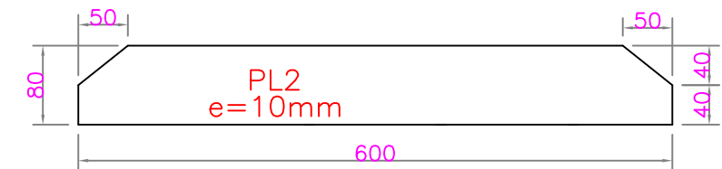
DETALLE PL2 ESCALA 1 : 7.5
