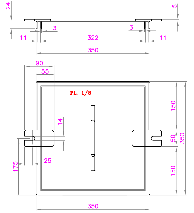
DETALLE DE TAPA ESCALA 1 : 2,5
