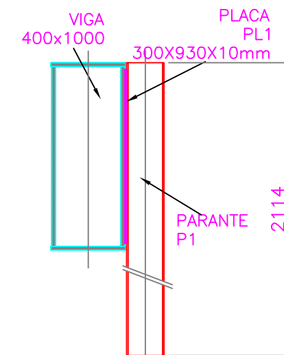
SOPORTE PARANTE P1 CANT: 2 UNIDADES ESCALA 1 : 30
