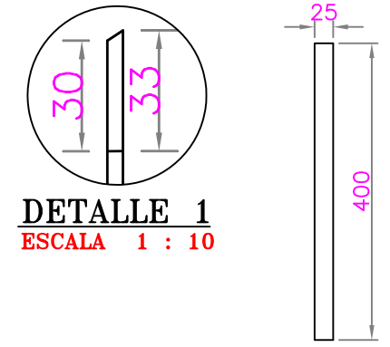
NERVIO (Cant. 4u) ESCALA 1 : 10
