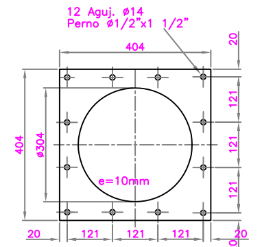
DETALLE BRIDA TIPO ESCALA 1 : 15 CANT: 1 U
