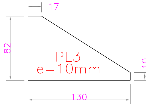
DETALLE PL3 CANT: 4 UNIDADES ESCALA 1 : 2.5
