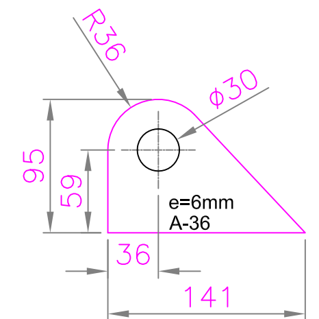
DETALLE DE OREJA CANT: 3 UNIDADES ESCALA 1 : 4
