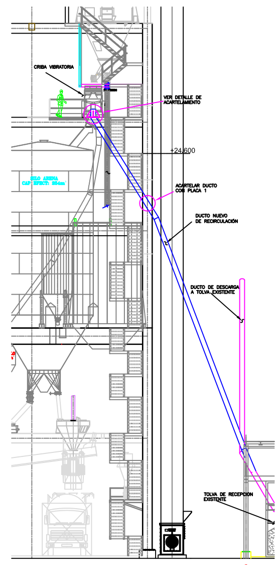
VISTA FRONTAL DUCTO ESCALA 1 : 125
