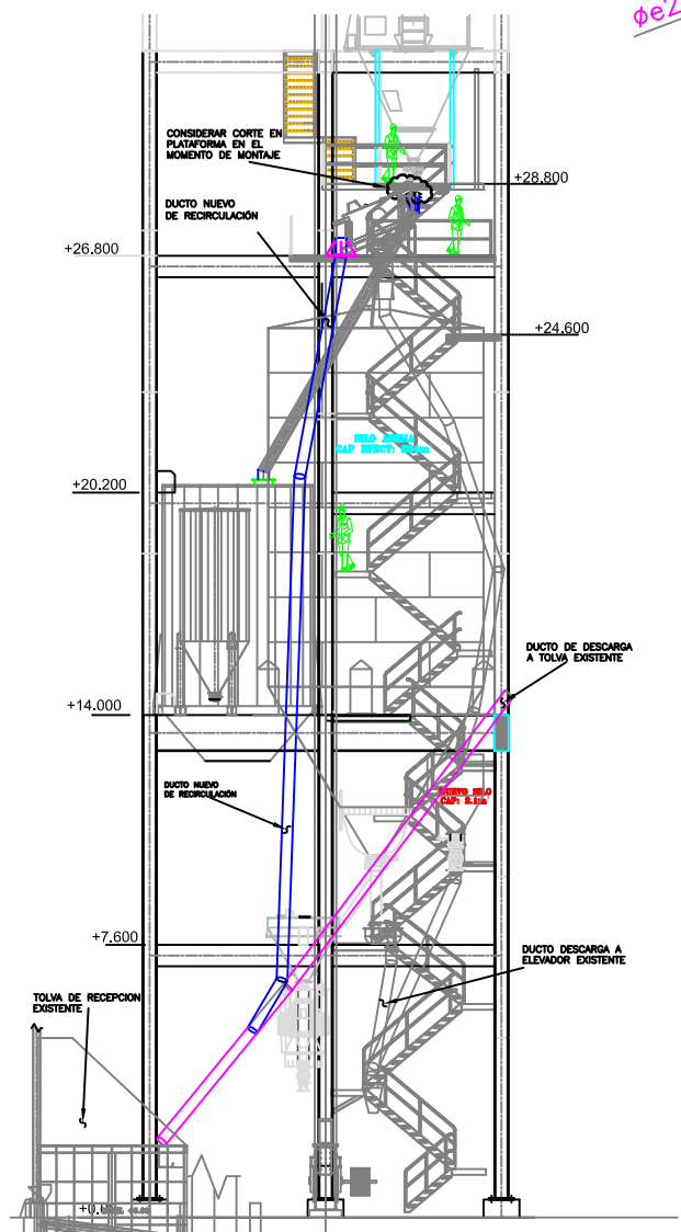
VISTA LATERAL DUCTO ESCALA 1 : 125
