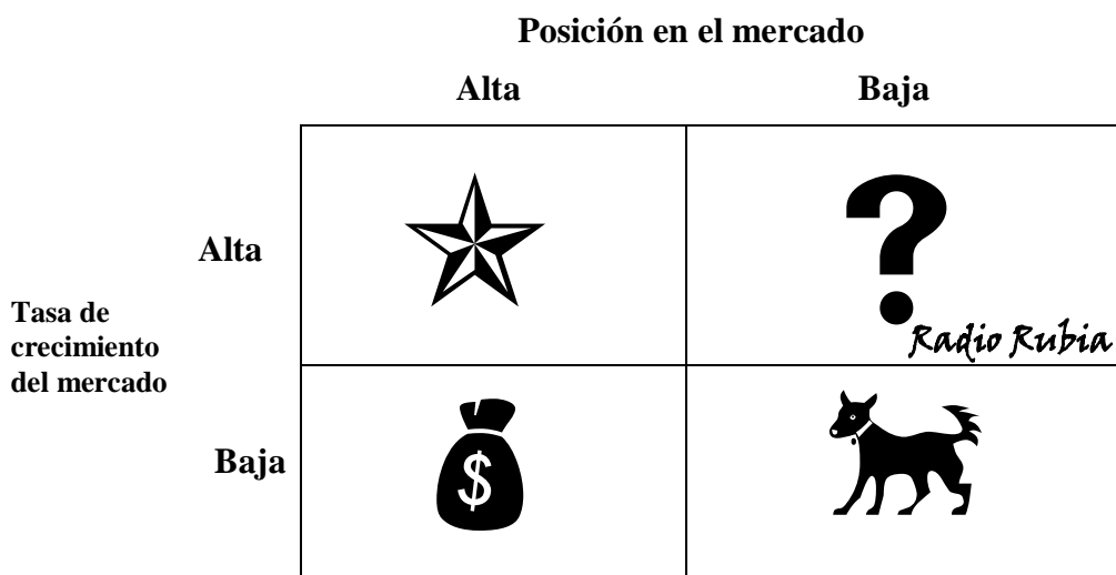
Figura 5.2. Matriz B.C.G
