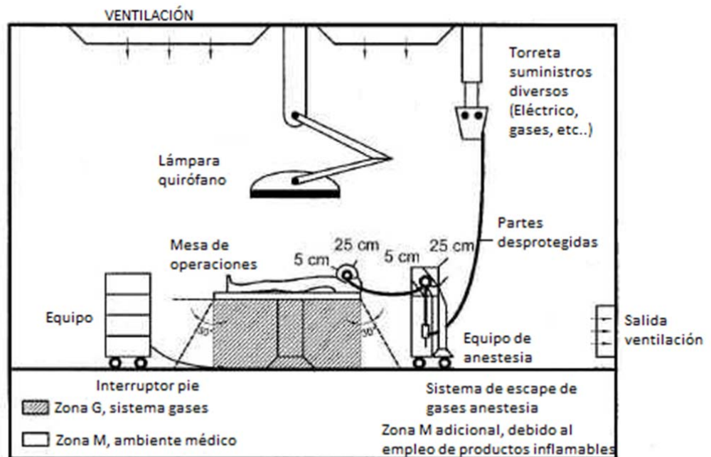
Figura. 2.4 Zonas con riesgo de incendio o explosión en el quirófano.
