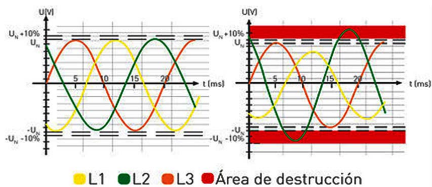
Figura. 1.1 Gráfica de una sobretensión permanente.
