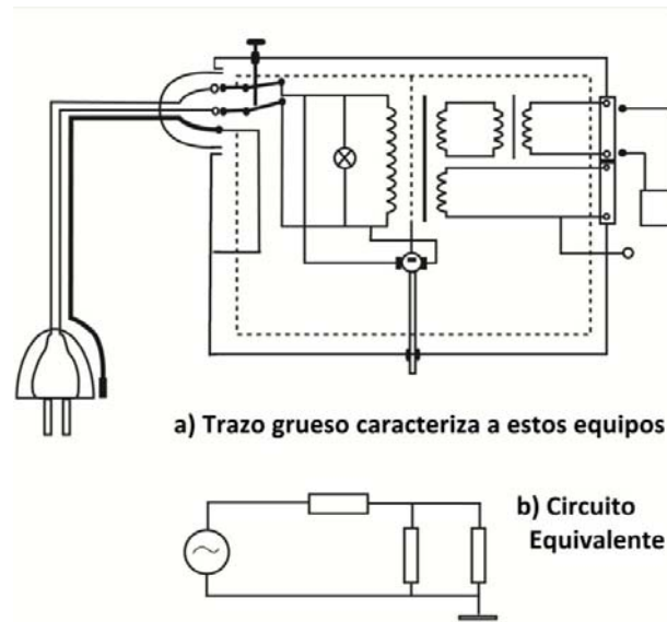
Figura. 1.11 Equipo clase I
