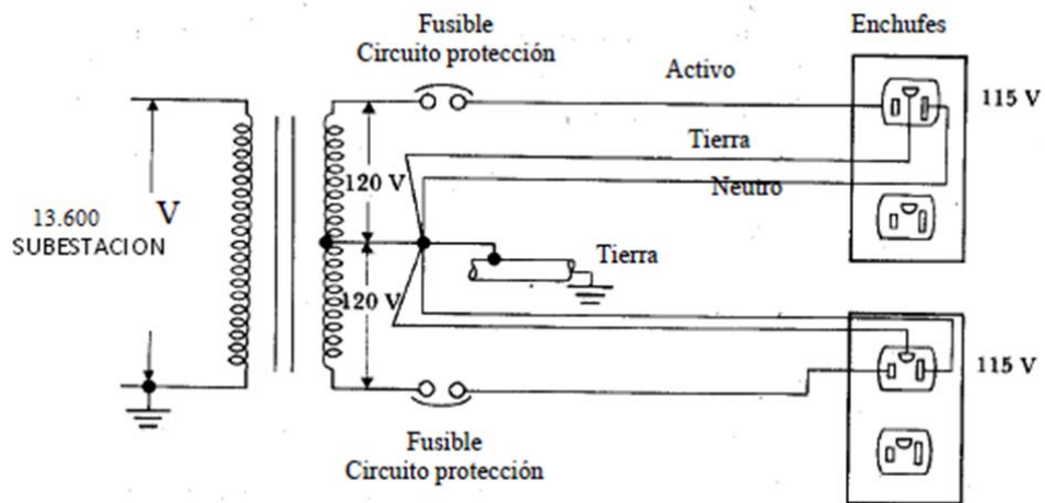
Figura. 1.10 Los tomacorrientes y la toma de tierra.
