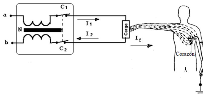
Figura. 1.7 Persona conectada a tierra en contacto con el circuito.
