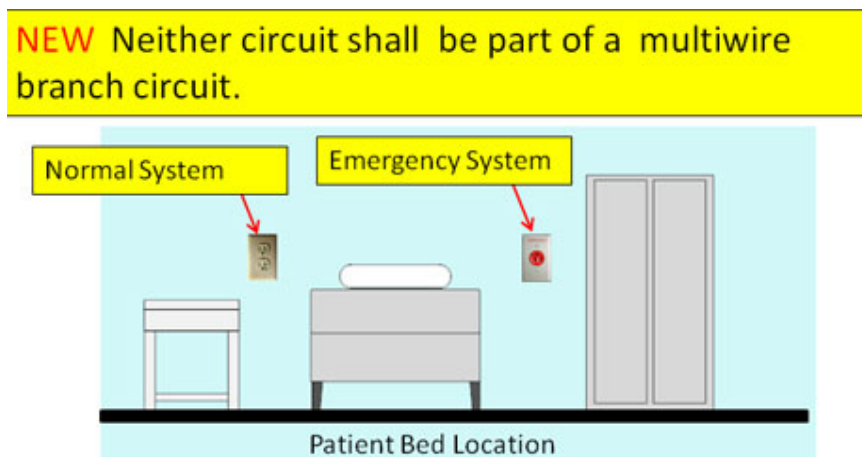
Anexo Figura 4. Tomacorrientes ubicados en las cercanías de las camas de pacientes.
