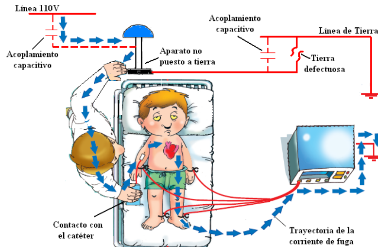
Figura. 1.6 Caso común que conduce a un microshock
