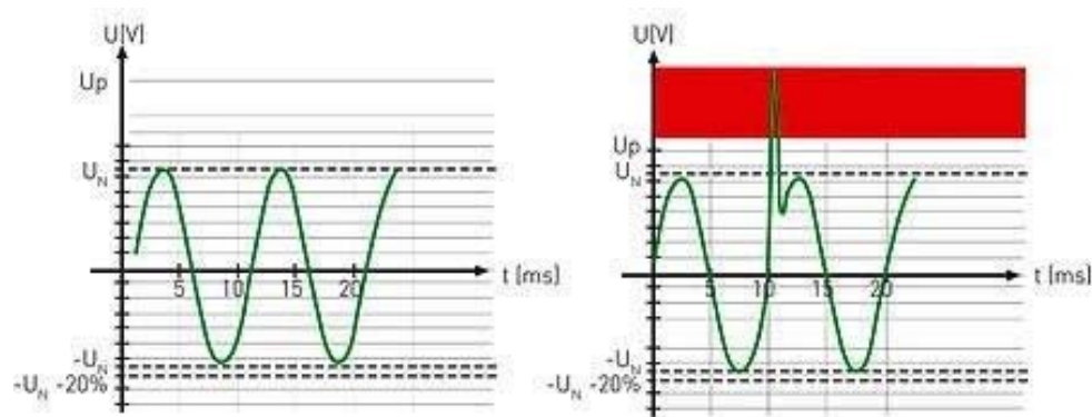
Figura. 1.2 Gráfico de una sobretensión transitoria.
