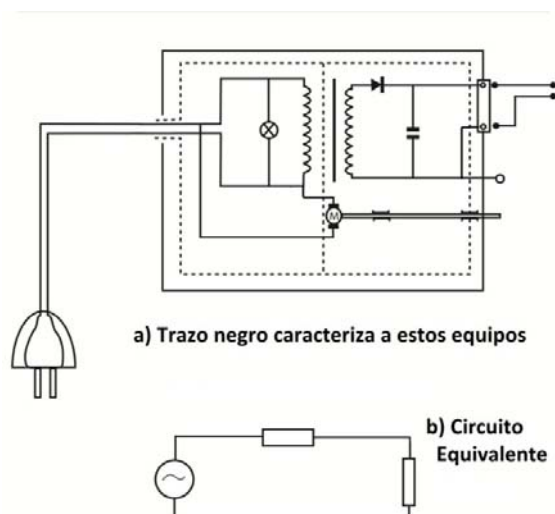
Figura. 1.13 Equipo clase III
