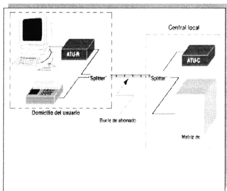
GRAFICO 5.6 CONEXIÓN ADSL
