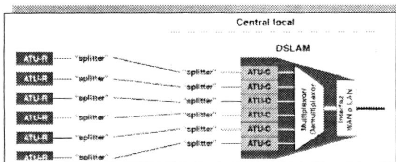
GRAFICO 2.5 ESTRUCTURA DE UN ARMARIO DSLAM
