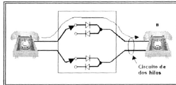
GRÁFICO 1.2 CONEXIÓN TELEFONÍA FIJA
