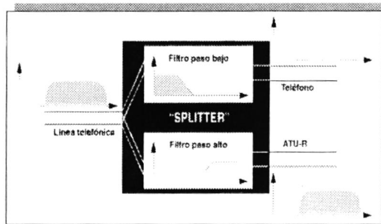
GRAFICO 5.7 FUNCIONAMIENTO DEL SPLITTER
