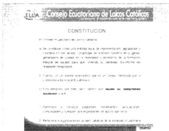
Figura 4-6 Página “Constitución”
