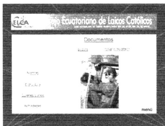
Figura 4-11 Página "Documentos"
