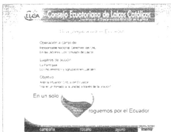
Figura 4-17 Página "Plegaria"
