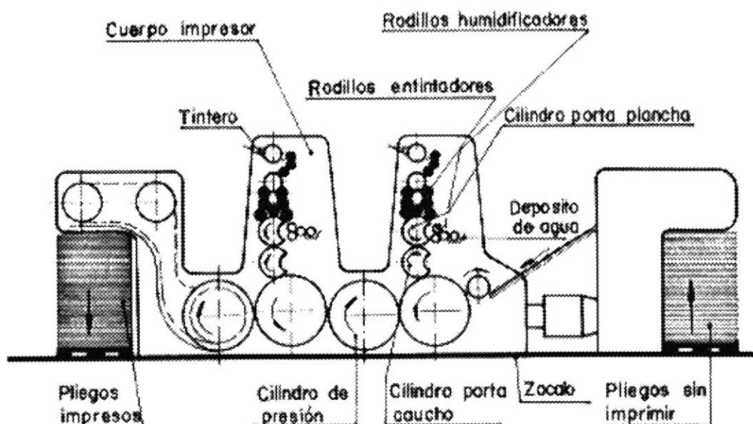
Figura 2.1 : Sistema de impresión offset
