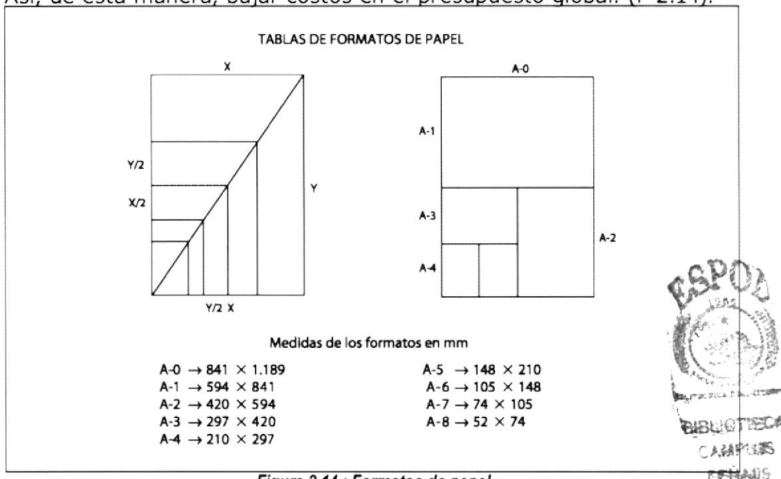
Figura 2.14 : Formatos de papel
