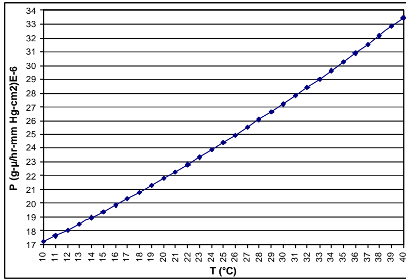
FIGURA 3. PERMEABILIDAD VS. TEMPERATURA DE TRICAPA A
