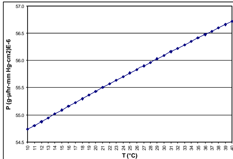
FIGURA 7. PERMEABILIDAD VS. TEMPERATURA DE TRICAPA E
