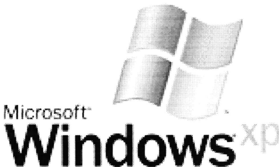
Fig.3.2.1. Sistema Operativo
