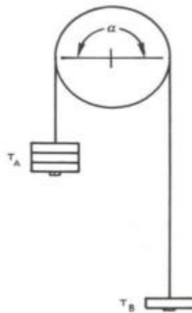
FIGURA 3.4 Tensiones T_a y T_b
