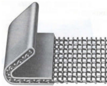
Figura 3.23 Gancho Tipo 2 con Platina Metálica.
