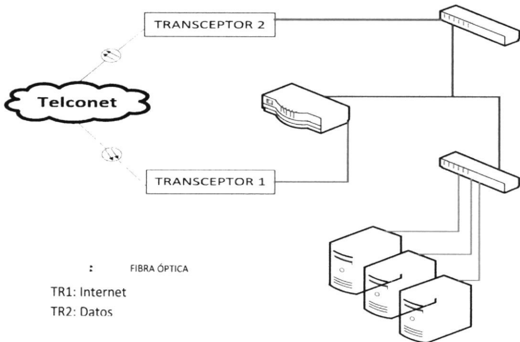
Gráfico 3-4: Transceptores y Conexión
