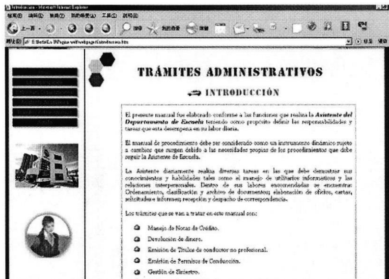
Fig. 4.21 Página “Introducción”
