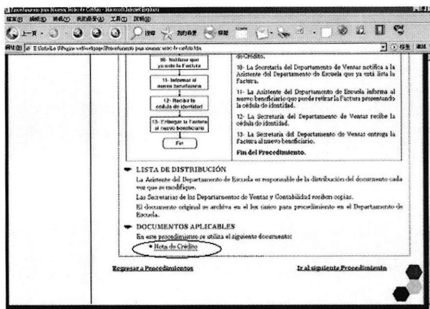
Fig. 4.28 Documentos Aplicables
