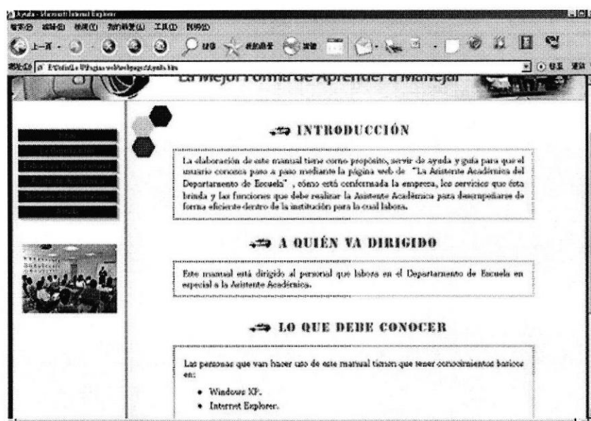
Fig. 4.29 Página "Ayuda"
