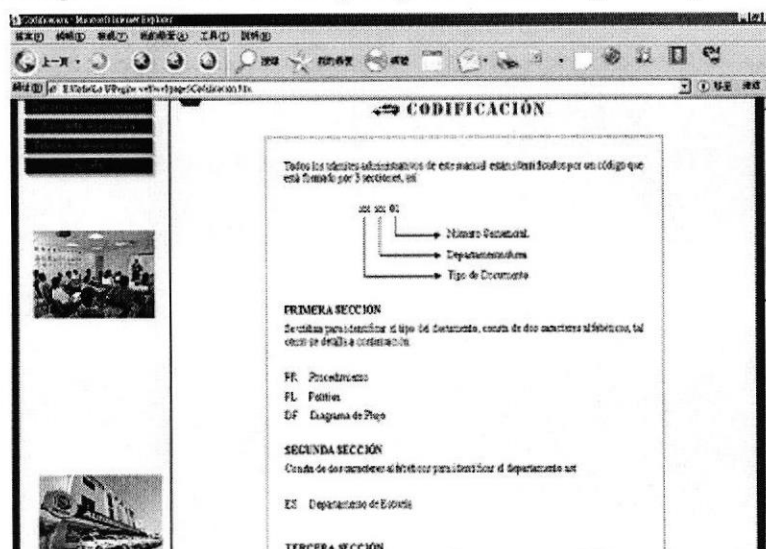
Fig. 4.23 Página “Codificación”
