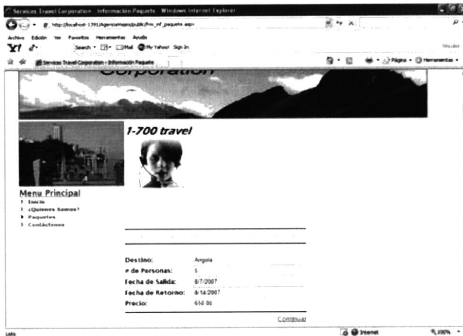
Figura 9-7: Paquete seleccionado.
