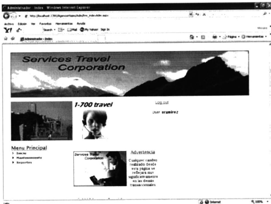
Figura 8-3: Inicio
