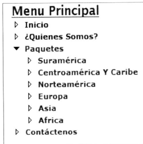
Figura 7-4: Menú Paquetes
