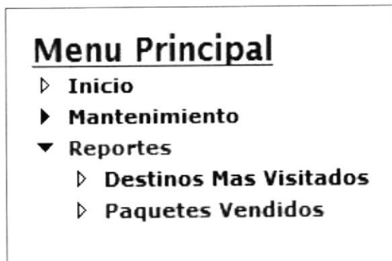
Figura 8-15: Menú Reportes
