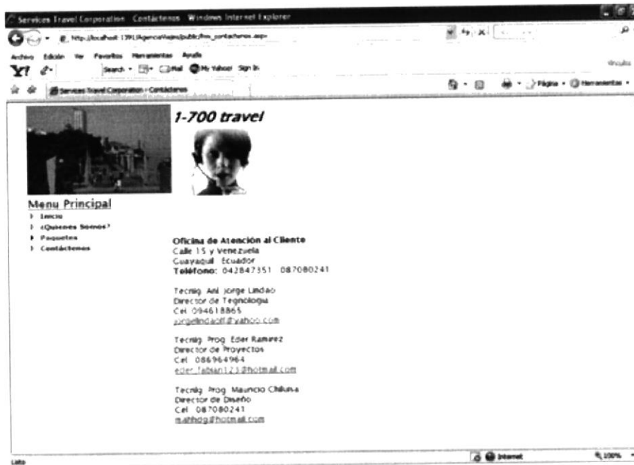
Figura 7-10: Contáctenos
