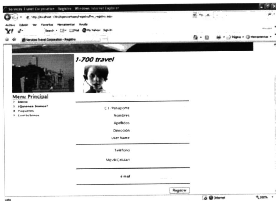
Figura 7-8: Registro usuarios
