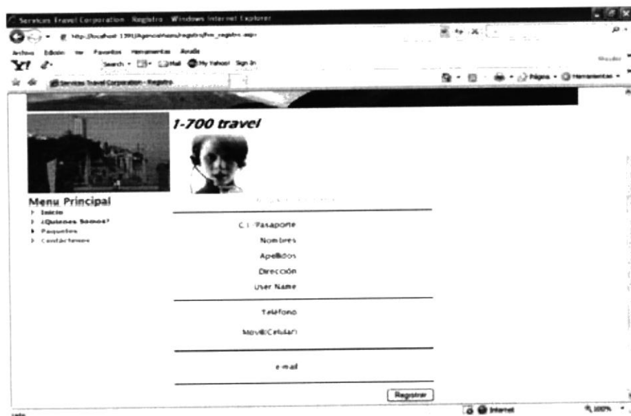
Figura 9-9: Registro usuarios
