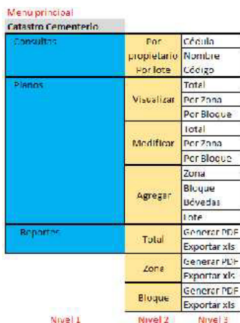
Figura 27 Menú principal requerido en componente ACL
