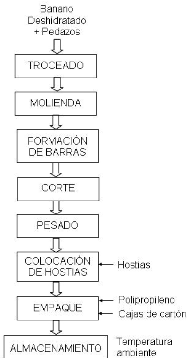
FIGURA 3.1 DIAGRAMA DE FLUJO DE ELABORACIÓN DE BARRAS DE BANANO DESHIDRATADO
