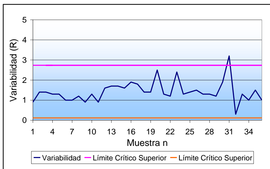
GRÁFICO 3.13 VARIABILIDAD DEL PROCESO
