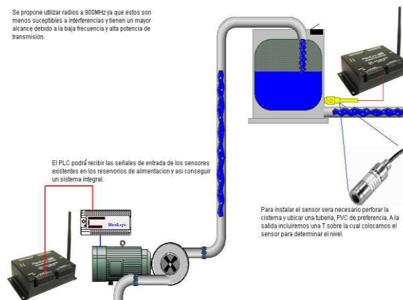
Figura 6. Estación reguladora de presión
