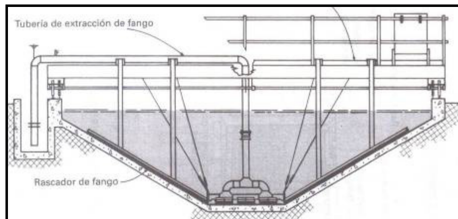
Figura 1.6 Tanque de Sedimentación de paredes inclinadas (13) .
