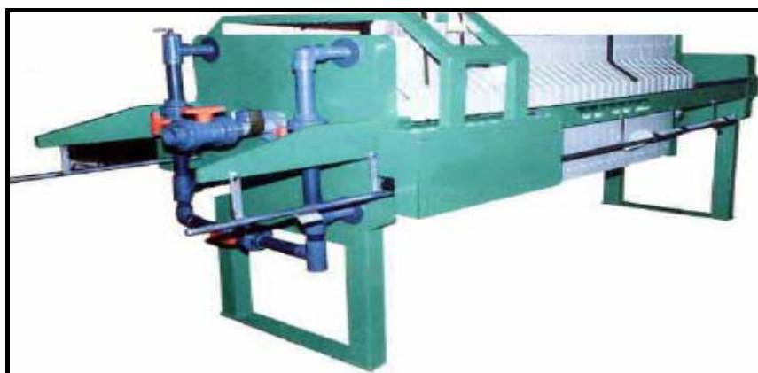
Figura 1.17 Filtro prensa (29) .
