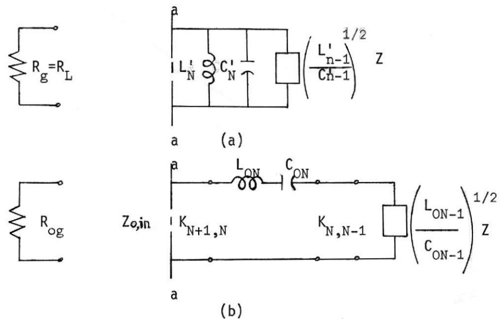
Fig. 1-8 Ultima sección del filtro para N impar.
