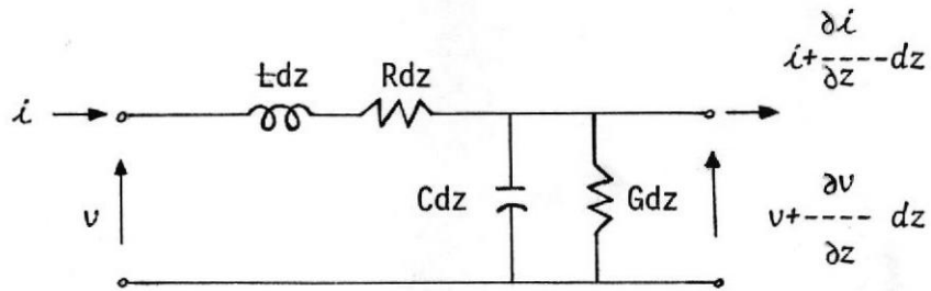
Fig. A-1 Circuito equivalente de una longitud diferencial de línea de transmisión.
