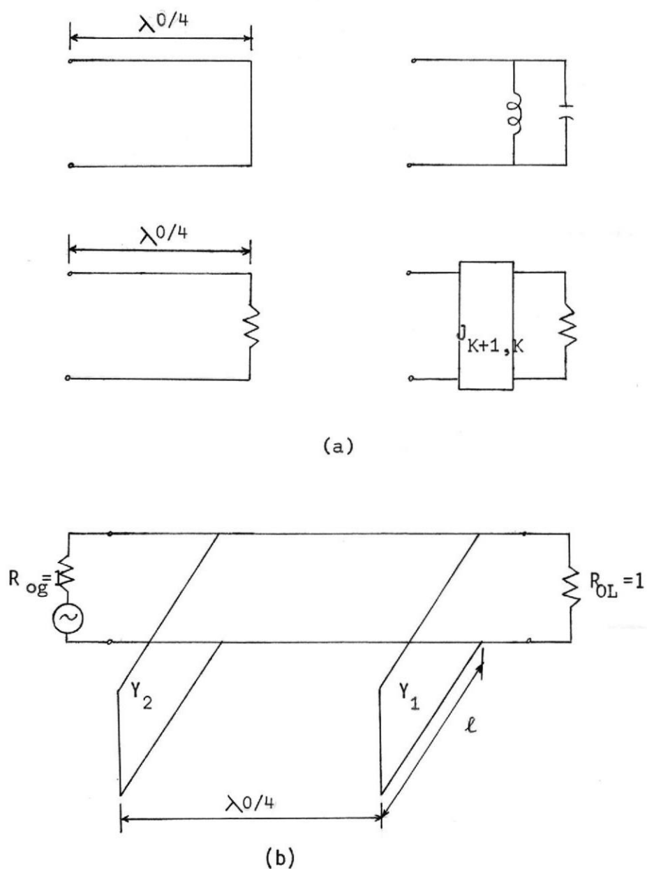
Fig. 2-1 Filtro de línea de transmisión usando fragmentos acoplados a un cuarto de onda.
