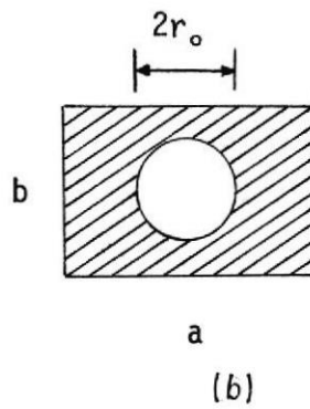
Fig. B-1 Elementos inductivos paralelos; (a) diafragma simétrico; (b) pequeña apertura circular.
