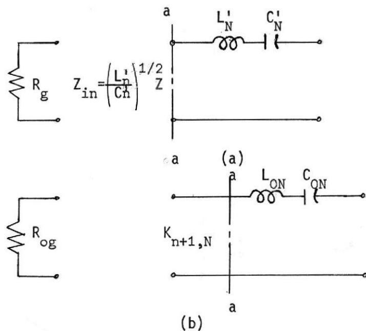
Fig. 1-7 Ultima sección del filtro para N par
