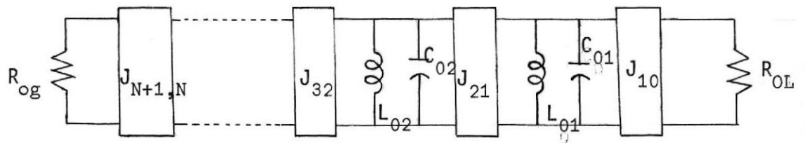
Fig. 1-9 Red de filtro equivalente obtenida por uso de inversores de admittancia.
