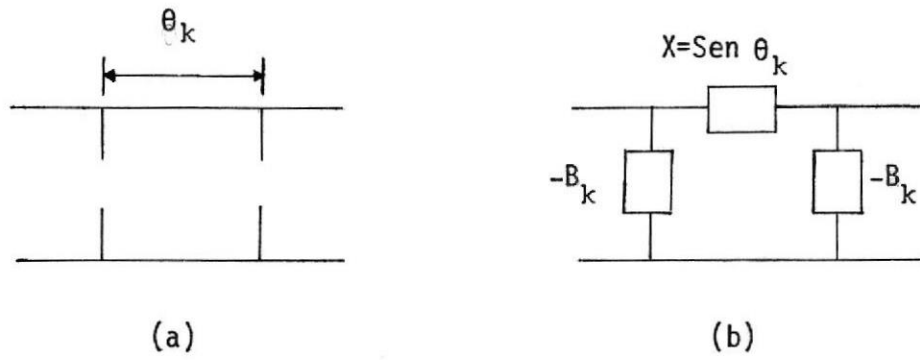
Fig. 2-4 Una cavidad de guía de onda y su circuito equivalente.
