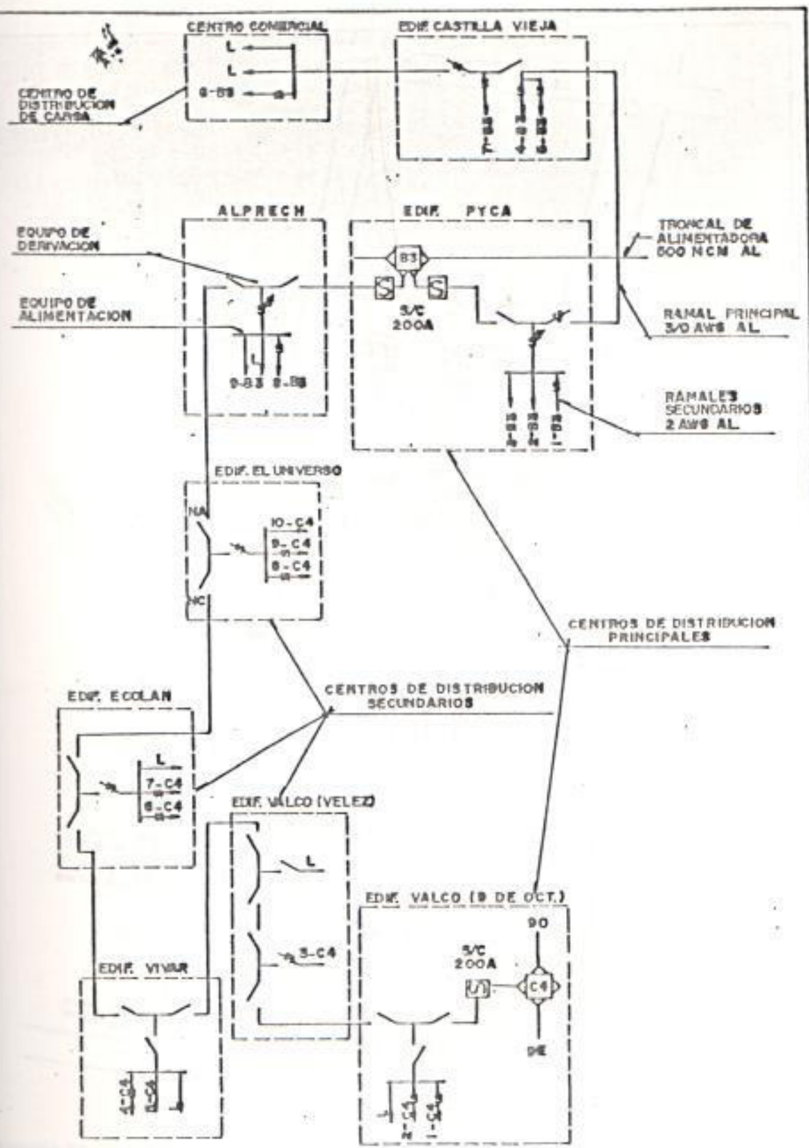
FIGURA 1.6. -- TIPOICO ARREGLO DE DISTRIBUCION DEL SISTEMA SUBTERRANEO.
