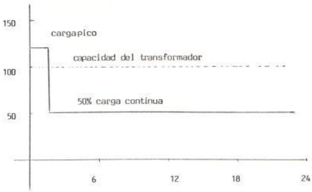
FIG. 5.2 CICLO DE CARGA CONTINUA
