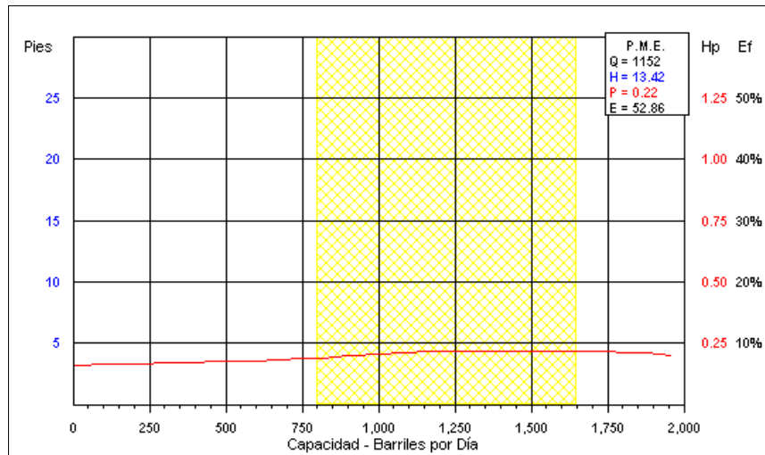
Fig. 4.3. Curva de la Potencia al Freno
