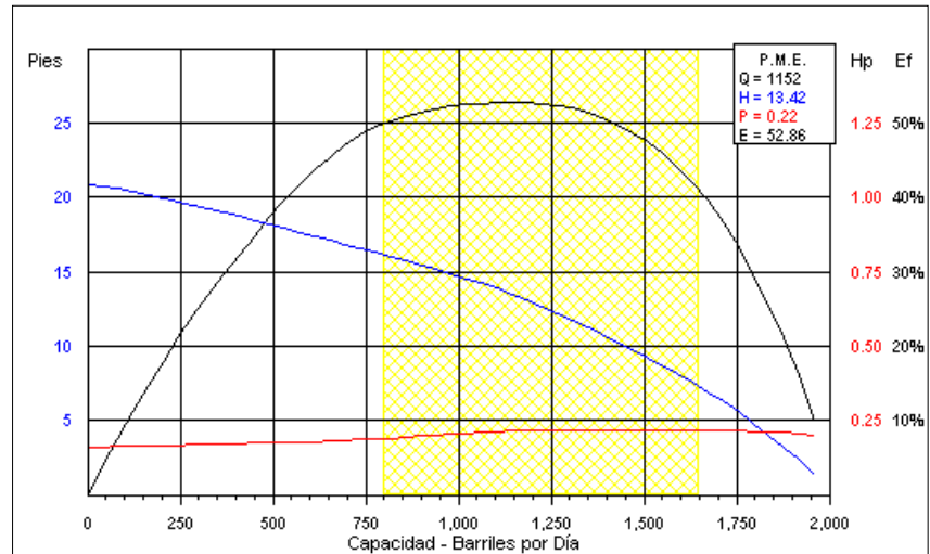
Fig. 4.2. Curvas de operación de una bomba electrosumergible
