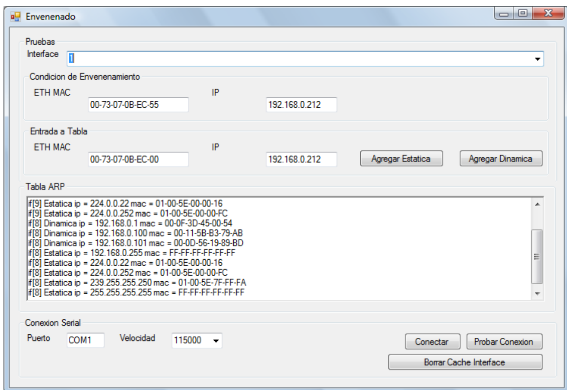
Figura 8: Pantalla de la implementación del atacado en entorno Windows
