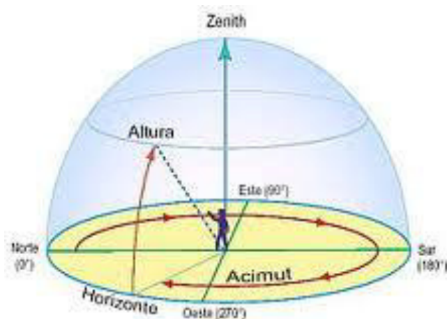
Figura N° 12 Esfera Celeste Local. 12
