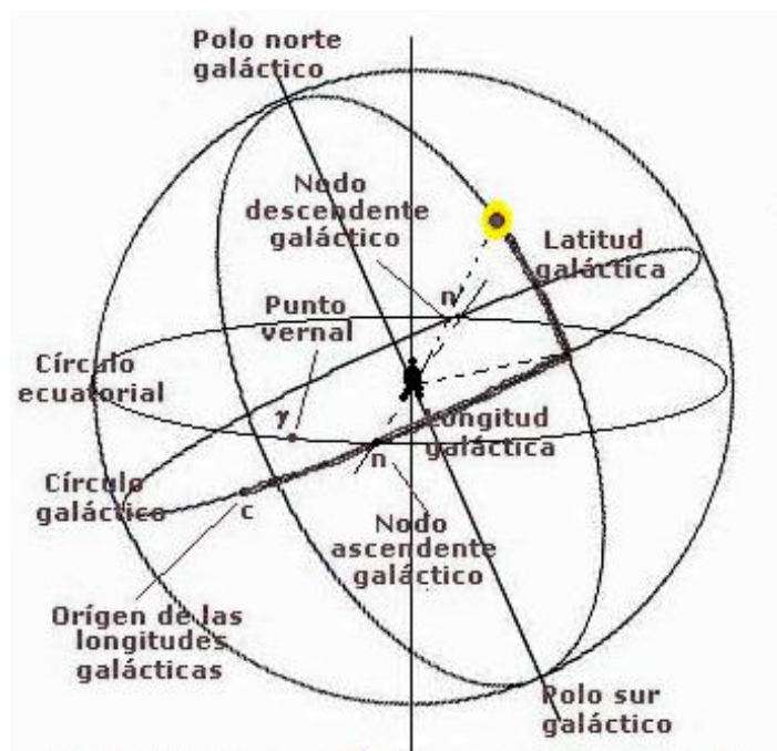
Figura Nº 25 Sistema de Coordenadas Galácticas 25
