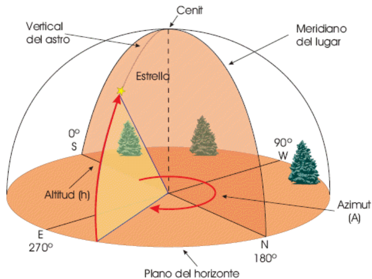
Figura N° 21 Coordenadas horarias. 21
