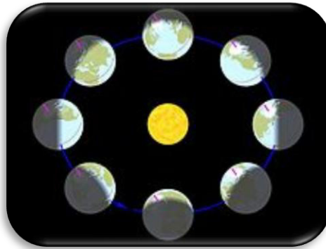
Figura N° 3 Movimiento de Traslación 3
