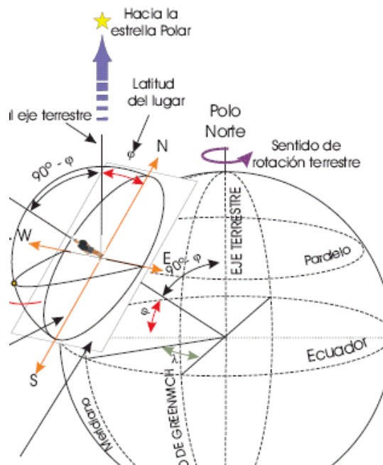
Figura N° 10 Representación de la longitud y la latitud de un determinado lugar de observación de un observador 10
