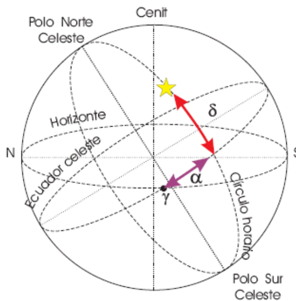
Figura N° 22 Coordenadas ecuatoriales absolutas. 22
