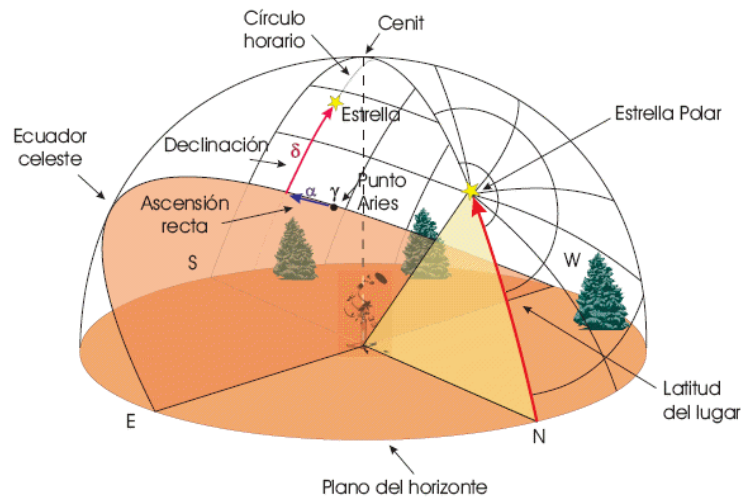
Figura N° 23 Coordenadas eclípticas. 23
