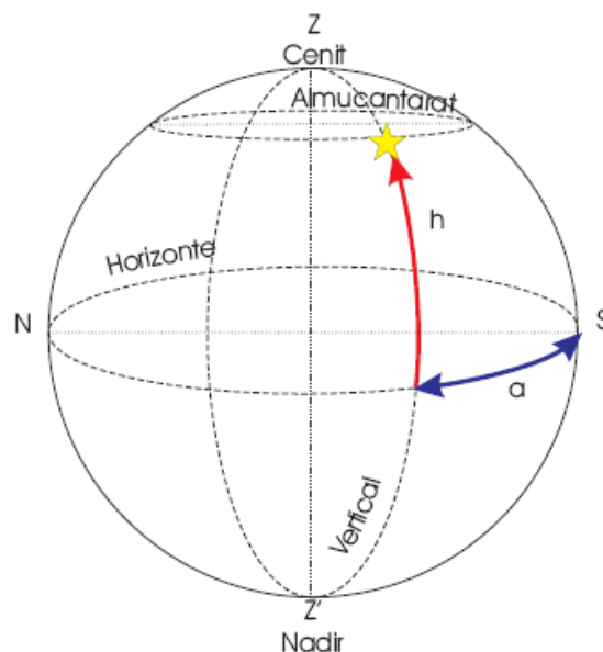
Figura Nº 20 Coordenadas astronómicas. 20
