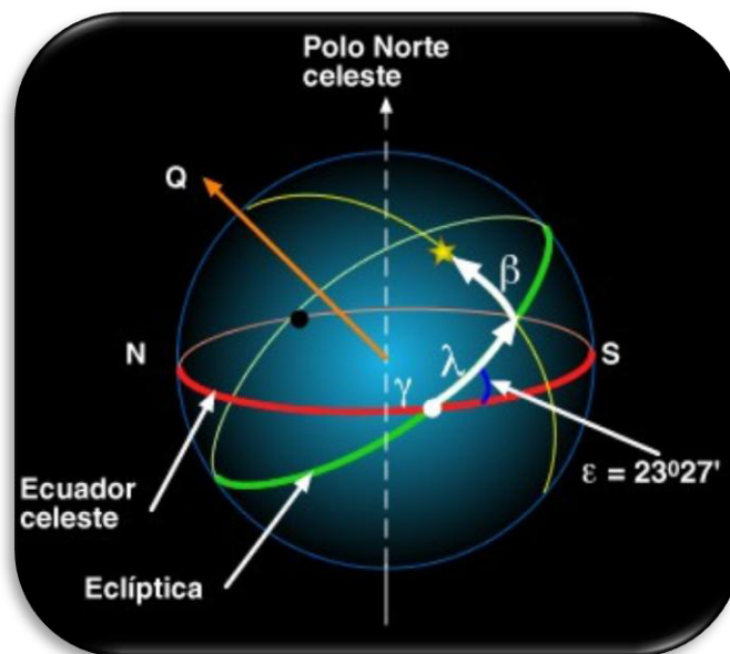
Figura N° 24 Utilización de las Coordenadas Eclípticas. 24
