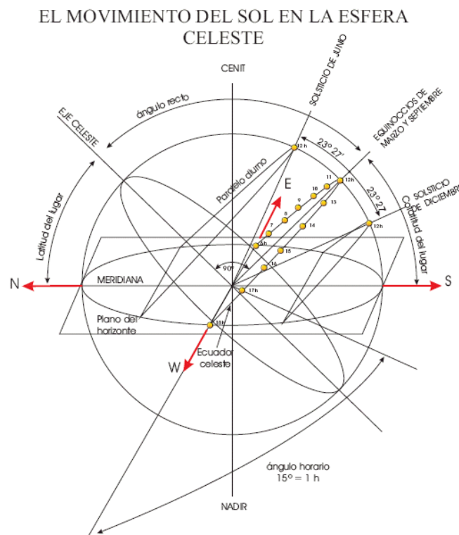
Figura N° 19 Movimiento del sol. 19
