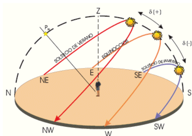
Figura N° 18 Movimiento del sol en la esfera celeste 18
