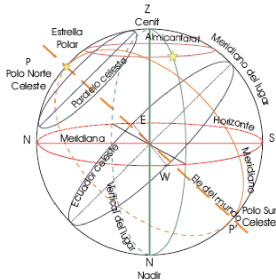
Figura N° 15 Sistema de Coordenadas 15
