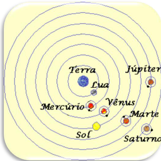
Figura N° 13 Sistema Geocéntrico. 13
