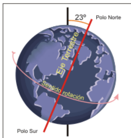
Figura N° 1 Movimiento de Rotación 1
