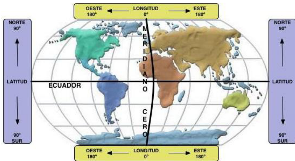
Figura N° 9 Coordenadas Geográficas. 9
