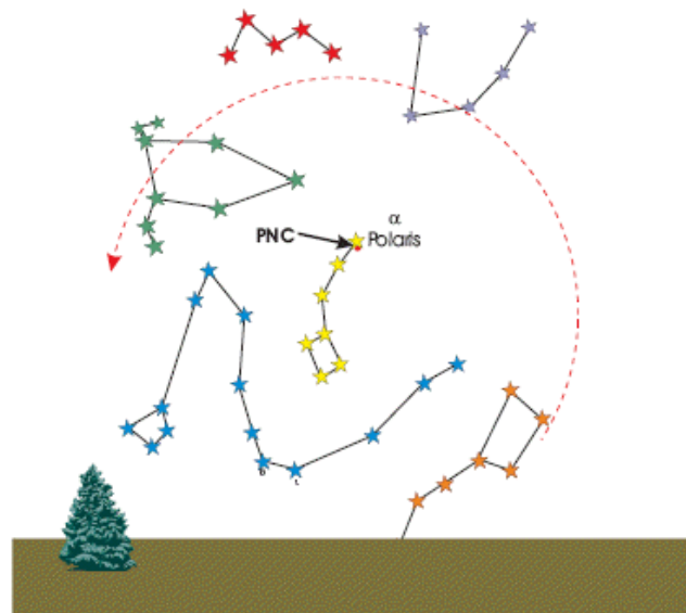
Figura N° 17 Movimientos aparentes de las constelaciones circumpolares alrededor del Eje del mundo o Polo Norte Celeste. 17
