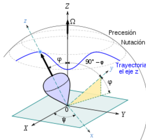
Figura N° 7 Caracterización del Movimiento de Nutación. 7
