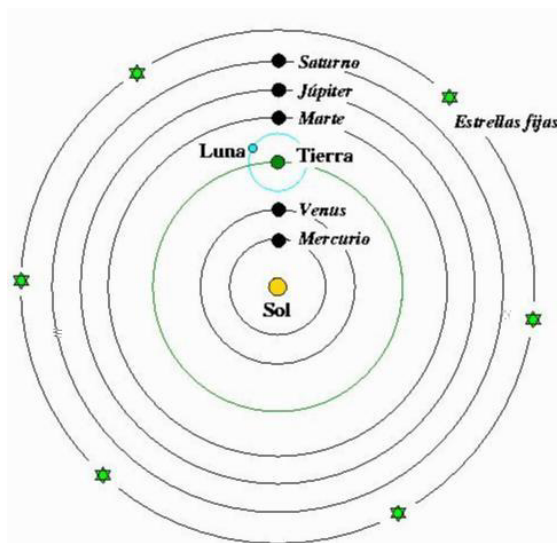
Figura N° 14 Sistema Heliocéntrico. 14
