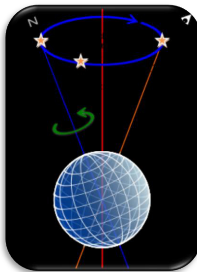
Figura N° 5 Angulo de Precesión 5
