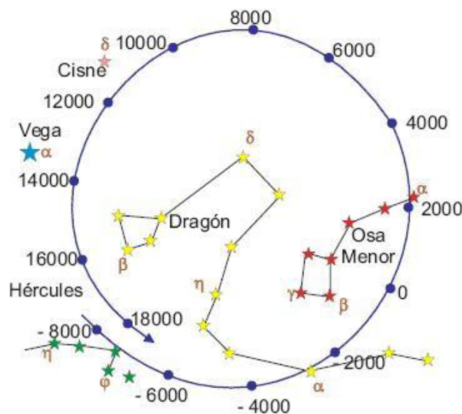
Figura N° 6 Movimiento de Precesión de la Tierra. 6
