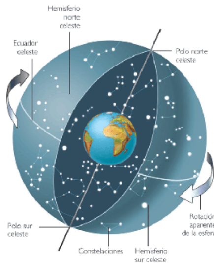
Figura Nº 2 Rotación de la Tierra en la Esfera Celeste 2
