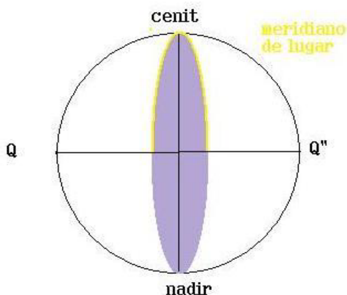
Grafico VII. Horario de lugar 13 .
