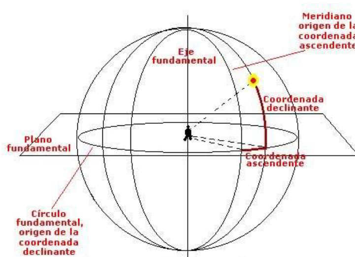
Gráfico III. Sistema de coordenadas astronómicas 6
