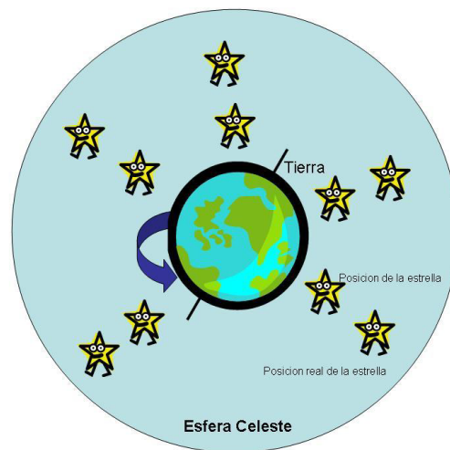
Figura I. La esfera celeste 1 .
