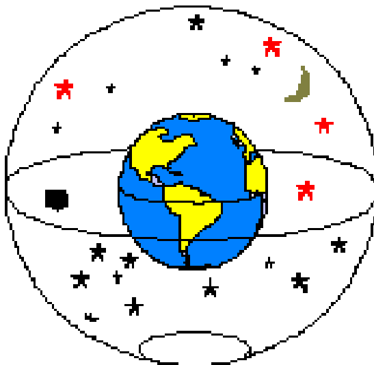
Figura V. La tierra y la esfera celeste 9 .
