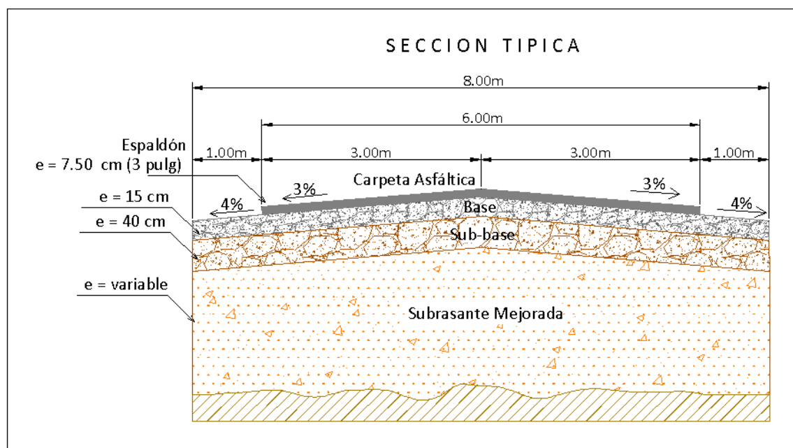
Figura 2-1. Sección típica del pavimento
