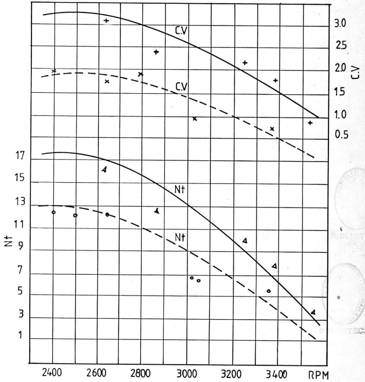
GRAFICO 5.1 CURVAS CARACTERISTICAS PARA GASOLINA Y GAS POBRE VELOCIDAD VARIABLE
