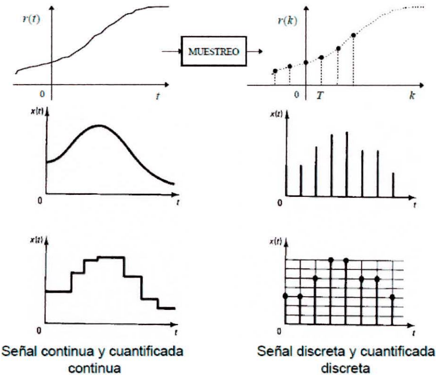
FIGURA 1.29: DISCRETIZACIÓN Y MUESTREO DE UNA SEÑAL
