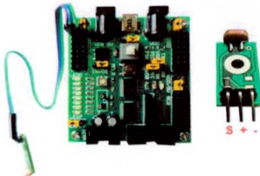
FIGURA 1.63: CONEXIÓN DEL MÓDULO LDR
