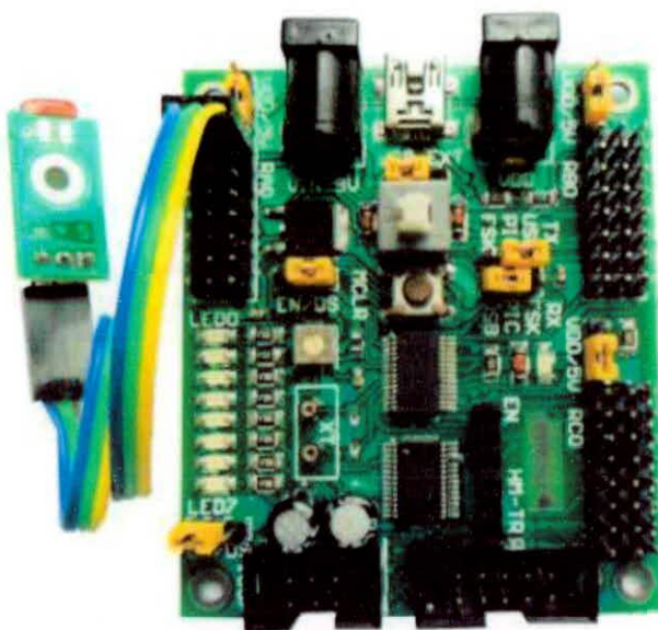
FIGURA 1.15: CONEXIÓN DEL SENSOR LDR
