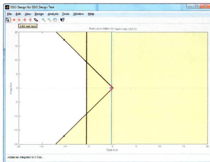
FIGURA 3.64: MODIFICACIÓN DE LA TRAYECTORIA DE LAS RAÍCES
