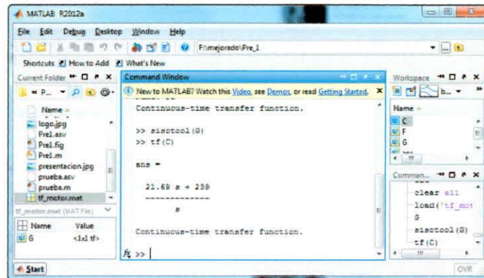
FIGURA 3.75: FUNCIÓN DE TRANSFERENCIA DEL CONTROLADOR
