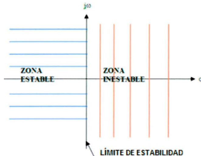
FIGURA 1.24: PLANO COMPLEJO S
