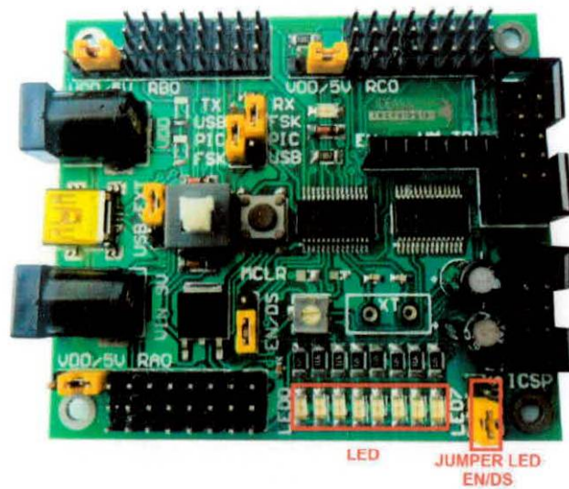
FIGURA 1.46: LEDS DEL MÓDULO MEI&T04
