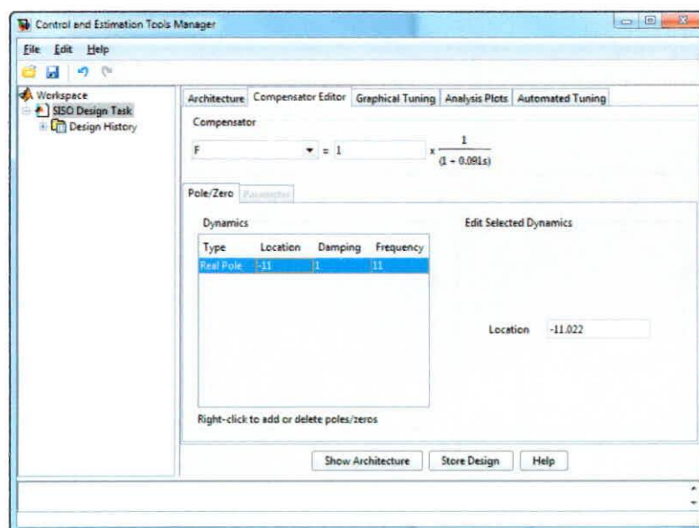
FIGURA 3.71: DISEÑO DEL PRE FILTRO
