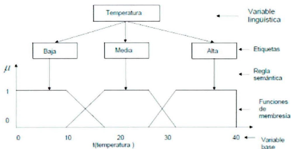
FIGURA 1.39: MODELO LINGÜÍSTICO
