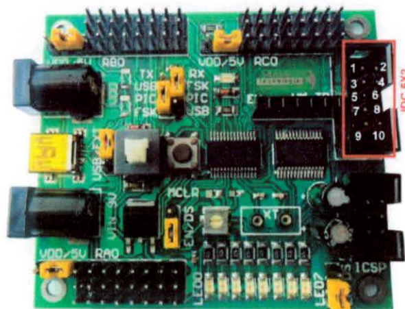
FIGURA 1.49: CONECTOR PARA CONTROL DE MOTORES DC DEL MÓDULO MEI&TO4
