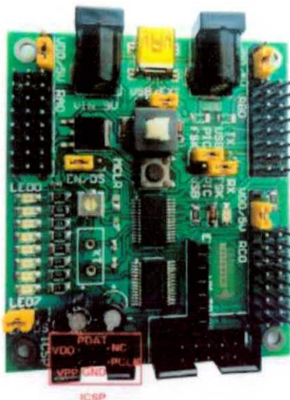
FIGURA 1.44: CONECTOR ICSP DEL MÓDULO MEI&T04
