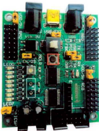
FIGURA 1.43: MCLR DEL MÓDULO MEI&T04
