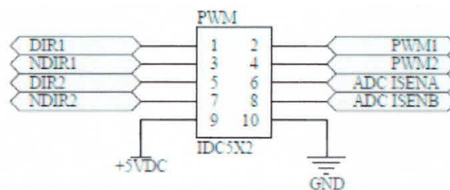
FIGURA 1.48: CONECTOR PARA CONTROL DE MOTORES DC
