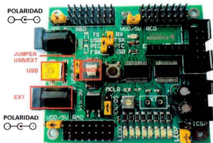
FIGURA 1.41: FUENTE DE ALIMENTACIÓN DEL MÓDULO MEI&T04
