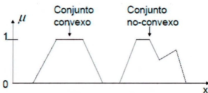
FIGURA 1.37: CONVEXIDAD
