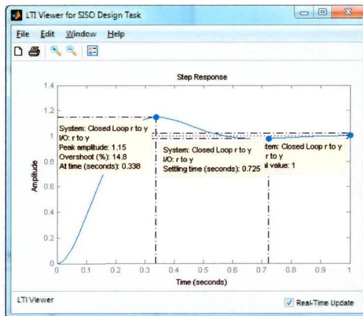
FIGURA 3.72: RESPUESTA DEL SISTEMA CONTROLADO
