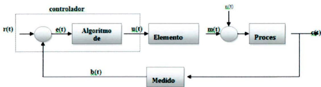
FIGURA 1.19: DIAGRAMA DE SISTEMA EN LAZO CERRADO
