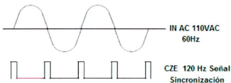
FIGURA 1.53: SEÑAL DE SINCRONIZACIÓN CRUCE POR CERO
