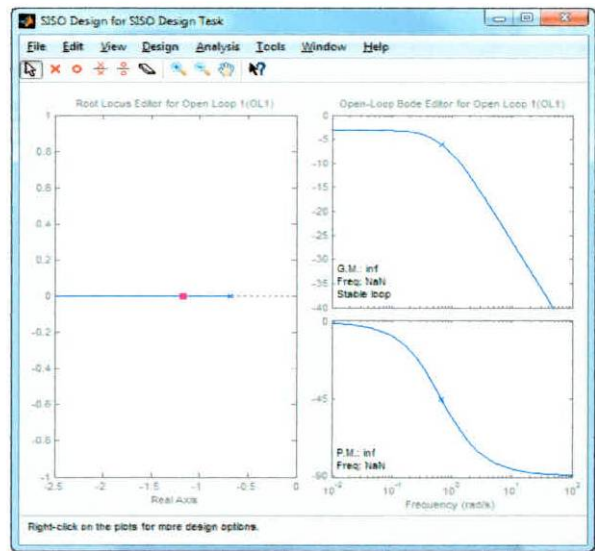
FIGURA 3.52: TRAYECTORIA DE LAS RAÍCES Y GRÁFICA DE BODE DEL SISTEMA
