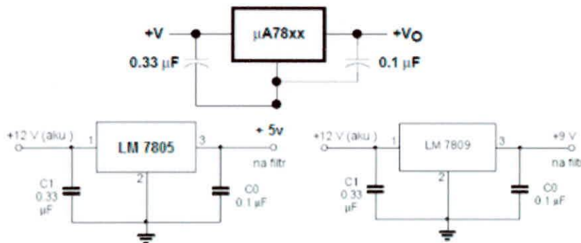
FIGURA 1.59: REGULADOR LM7805 – LM7809
