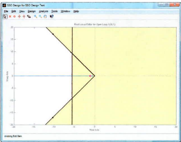
FIGURA 3.61: REQUERIMIENTO DE TIEMPO DE ESTABLECIMIENTO
