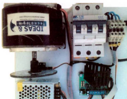
FIGURA 3.7: PLANTA CON MOTOR DC
