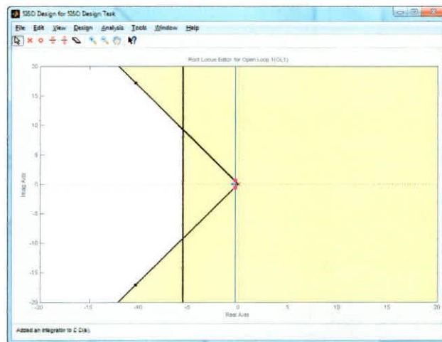
FIGURA 3.63: MODIFICACIÓN DE LA TRAYECTORIA DE LAS RAÍCES
