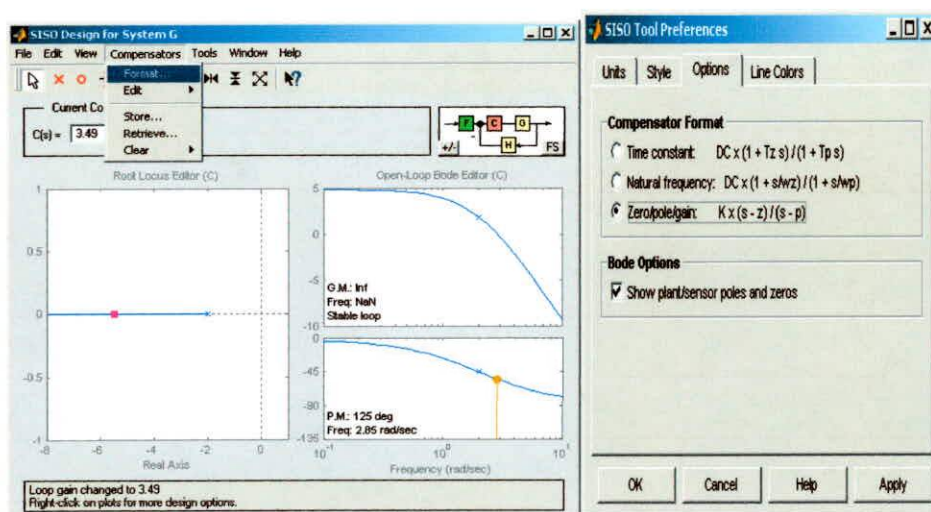
FIGURA 1.75: REPRESENTACIÓN FACTORIZADA DEL CONTROLADOR EN SISOTOOL
