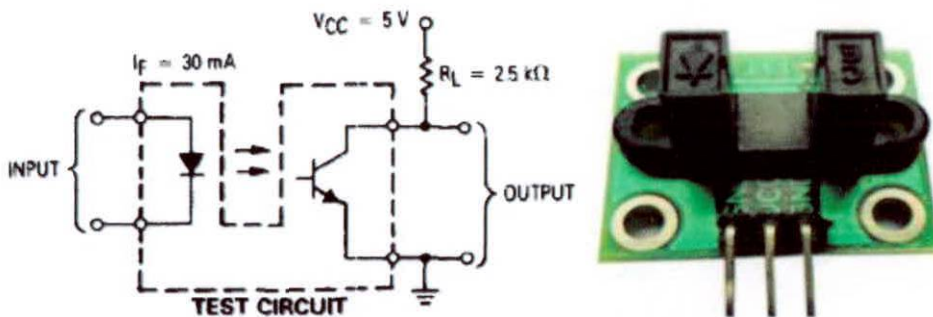
FIGURA 1.57: MÓDULO CON ENCODER MOC70T3
