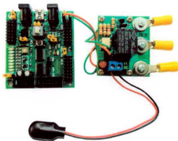
FIGURA 1.55: CONEXIÓN DEL MÓDULO DISPARADOR DE RELÉ
