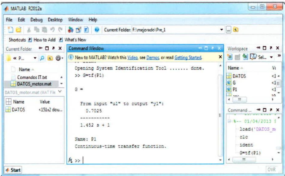
FIGURA 4.4: FUNCIÓN DE TRANSFERENCIA DEL MODELO DE ESTIMACIÓN
