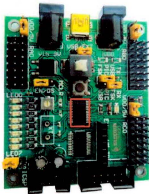
FIGURA 1.42: PIC 16F886 DEL MÓDULO MEI&T04
