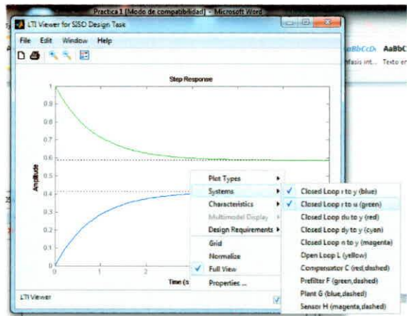
FIGURA 3.57: RESPUESTA ANTE UNA ENTRADA PASO
