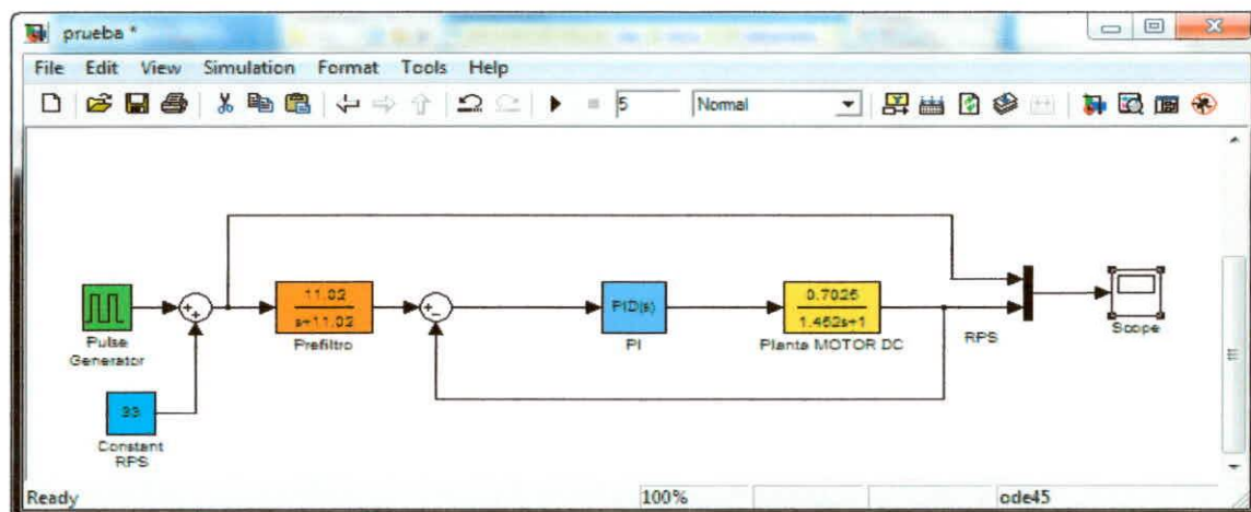
FIGURA 4.6: SISTEMA COMPLETO EN SIMULINK
