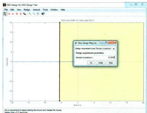
FIGURA 3.60: REQUERIMIENTOS DE SOBRE NIVEL PORCENTUAL
