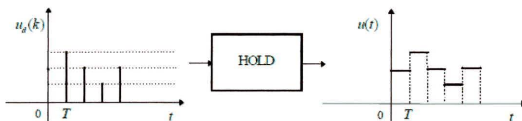
FIGURA 1.32: EFECTO HOLD
