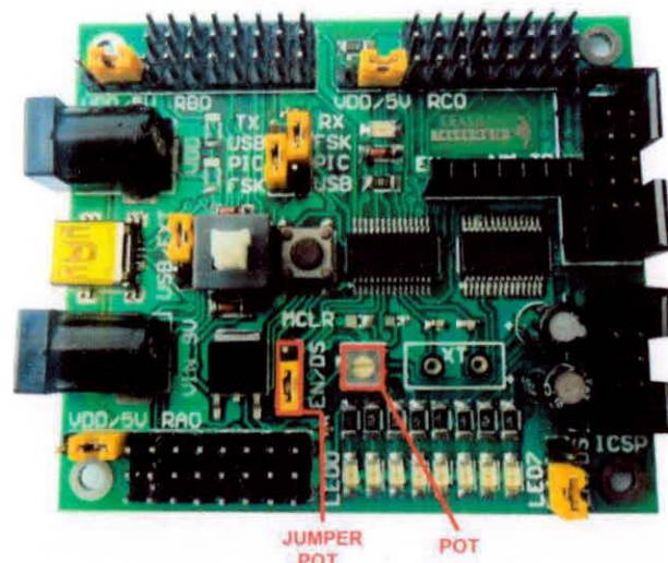
FIGURA 1.47: POTENCIÓMETRO DEL MÓDULO MEI&T04
