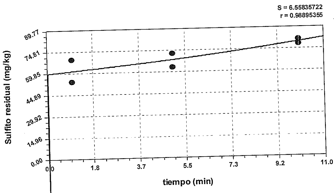
Figura 3.7 Modelo "Rational Function", 80 g/l y Temperatura de 12°C Elaborado por: Carmen Llerena.
