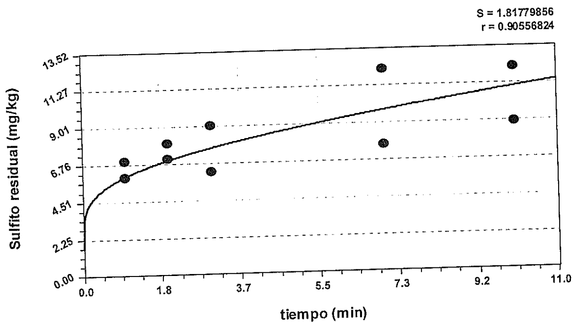
Figura 3.5 Modelo de Harris, 40 g/l y Temperatura de 5°C Elaborado por: Carmen Llerena
