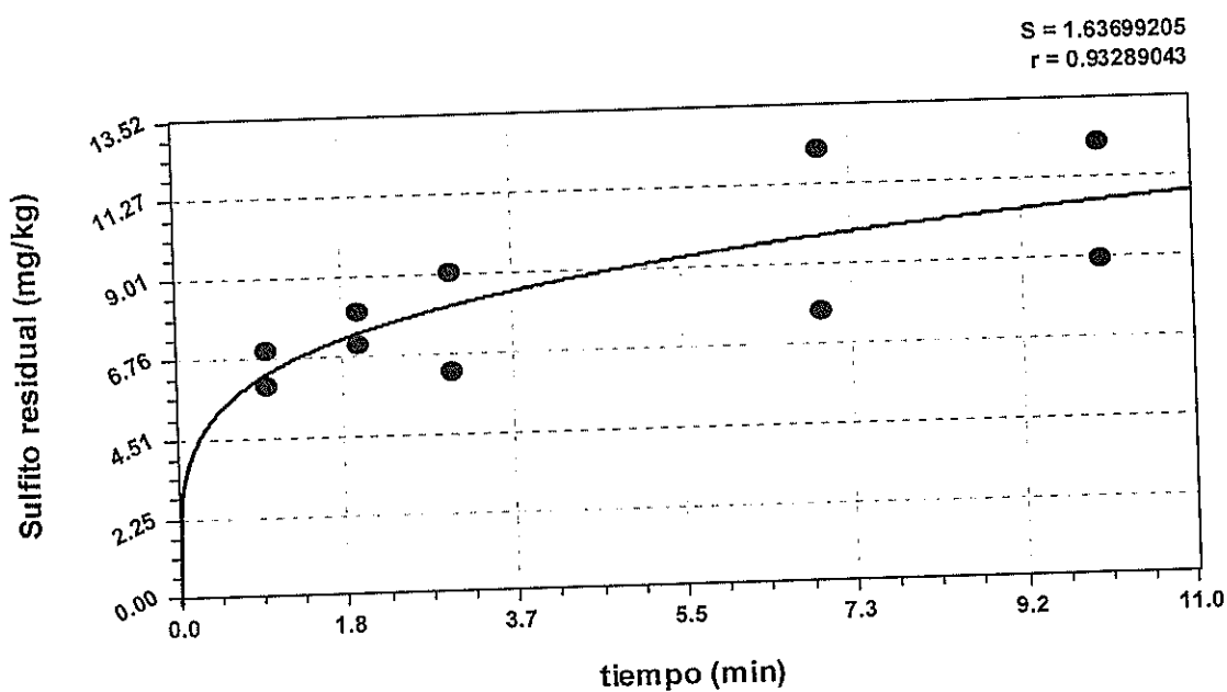
Figura 3.6 Modelo MMF, 40 g/l y Temperatura de 5°C Elaborado por: Carmen Llerena
