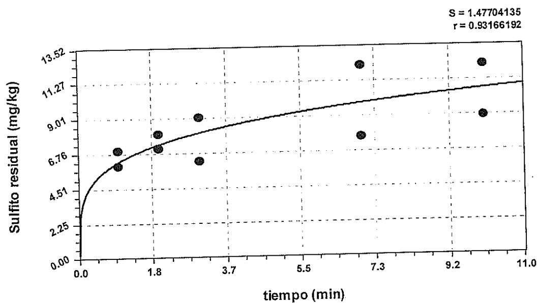
Figura 3.3 Modelo de Potencia, 40 g/l y Temperatura de 5°C Elaborado por: Carmen Llerena
