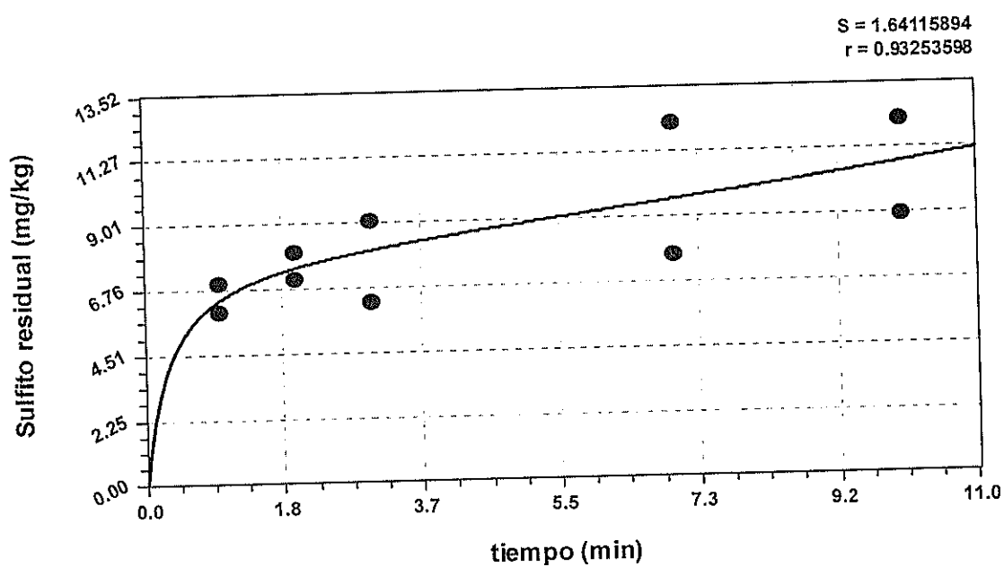
Figura 3.4 Modelo "Rational Function", 40 g/l y Temperatura de 5 °c Elaborado por: Carmen Llerena
