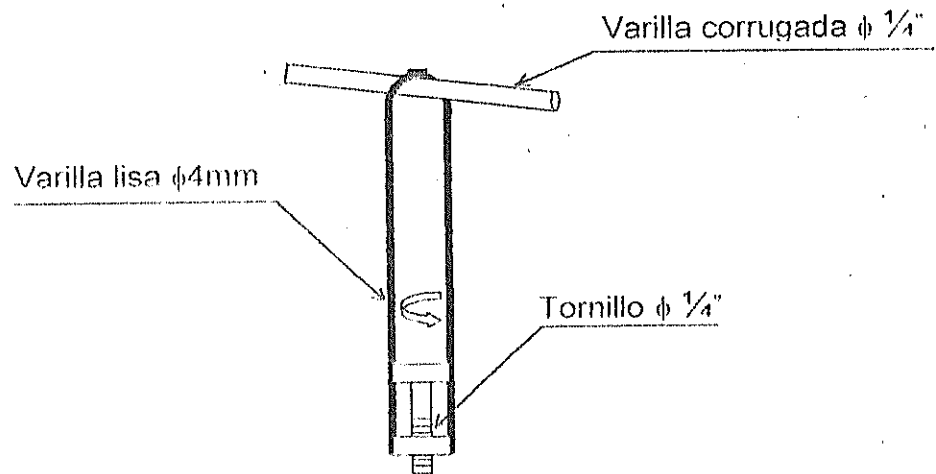
Figura 1.3.6: Herramienta para colocar los herrajes
